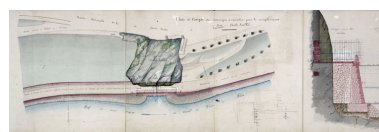
Remplacement du pont de la Porte taillée par un remblai perreyé. Dessins de détails du pont actuel et des ouvrages à y substituer [détail : ouvrages prévus], 1881. Phot. Yves Sancey, Phot. Paul Schoendoerffer IVR43_20062500349NUCA
