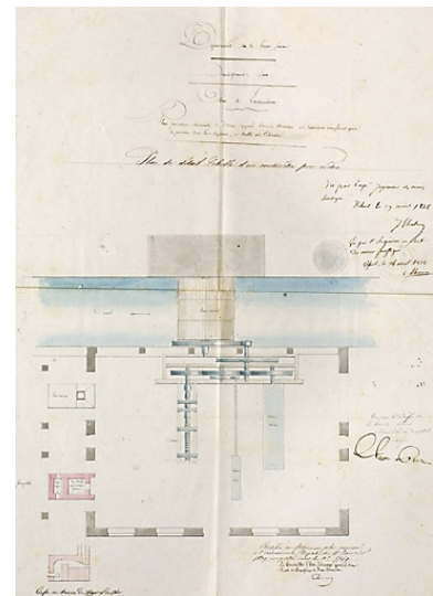
Plan présentant l'ensemble de l'usine appelée ancien martinet au laminoinf neuf ainsi que la position d'un four d'affinerie, et celle du cylindre. Phot. Jérôme Mongreville IVR43_20077000071NUCA
