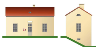
Schéma d'une maison éclusière de type Foucherot. Dess. Alain Morelière IVR26_20112100102NUDA
