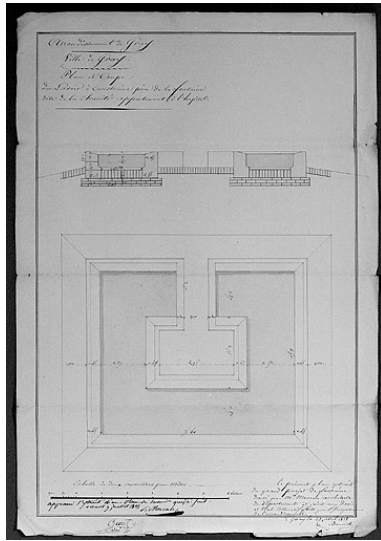
Plan et coupe du lavoir.
