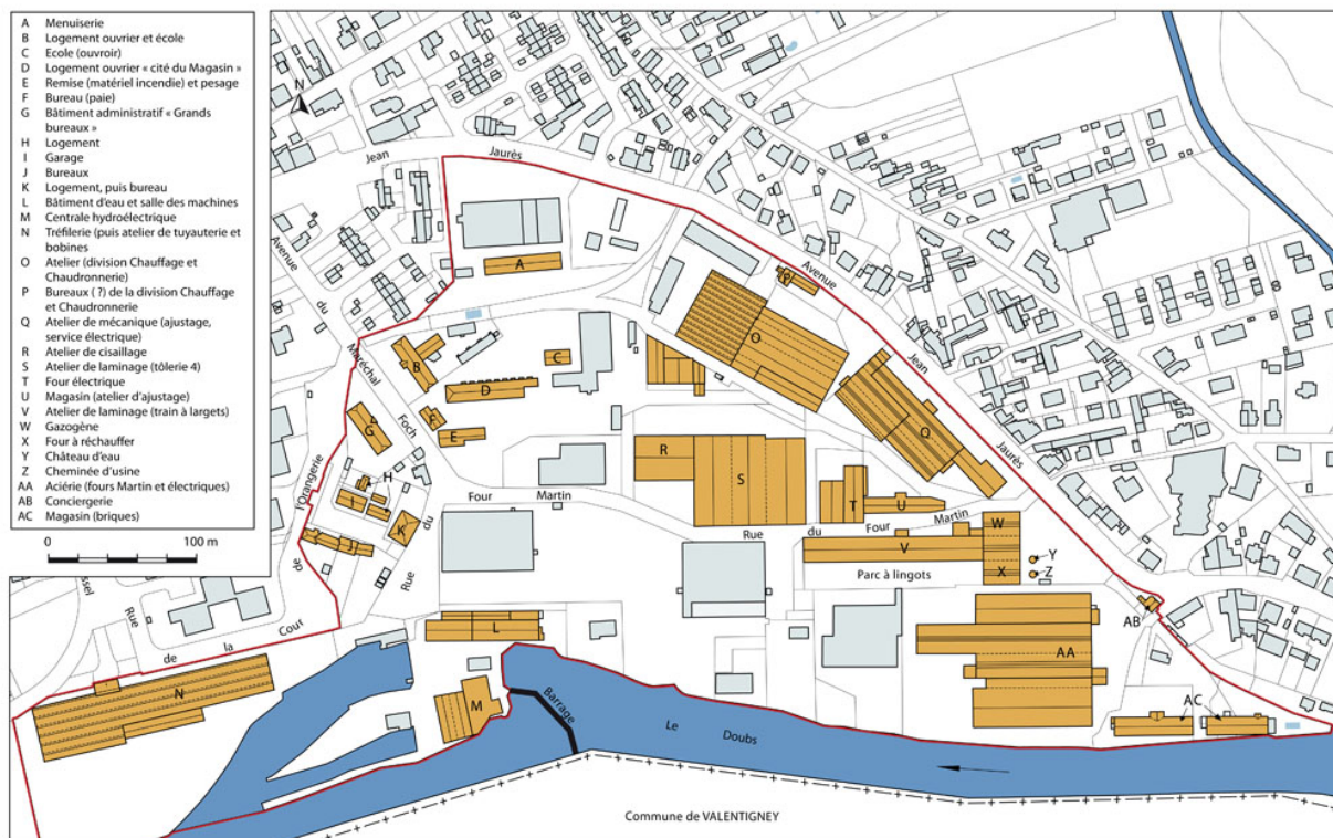
Plan-masse et de situation de l'usine métallurgique.
