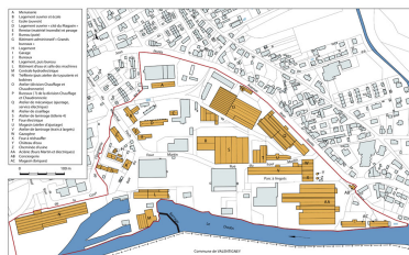
Plan-masse et de situation de l'usine métallurgique. Dess. Mathias Papigny IVR43_20132502534NUDA
