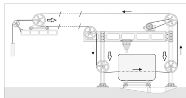
Schéma de fonctionnement d'une scie à fil hélicoïdal. Dess. André Céréza IVR43_20013900835NUDY
