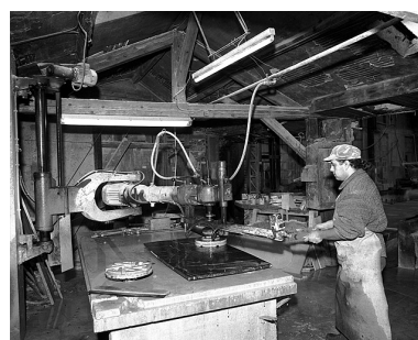
Usine de taille de matériaux de construction Célard, à Saint-Amour : le premier polissoir à genouillère.
