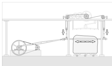
Schéma de fonctionnement d'un châssis de scie multilames. Dess. André Céréza IVR43_20013900836NUDY
