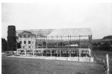
La raffinerie en construction depuis le sud. Phot. Emile Hérissé, Phot. Emile Hérissé IVR43_20077000474NUCA
