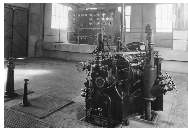
Centrale électrique. Le groupe turbo-alternateur Altshom. Phot. Emile Hérissé, Phot. Emile Hérissé IVR43_20077000464NUCA
