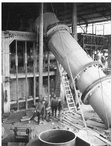
Mise en place du séchoir. Phot. Emile Hérissé, Phot. Emile Hérissé IVR43_20077000488NUCA
