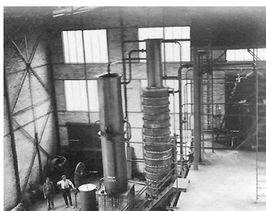
Intérieur de la raffinerie. Vue plongeante sur une colonne de distillation. Phot. Emile Hérissé, Autr. Emile (photographe) NEPASUTILISERHérissé IVR43_20077000479NUCA
