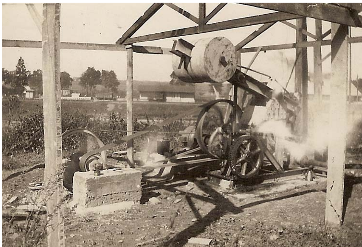
La pompe du forage.
