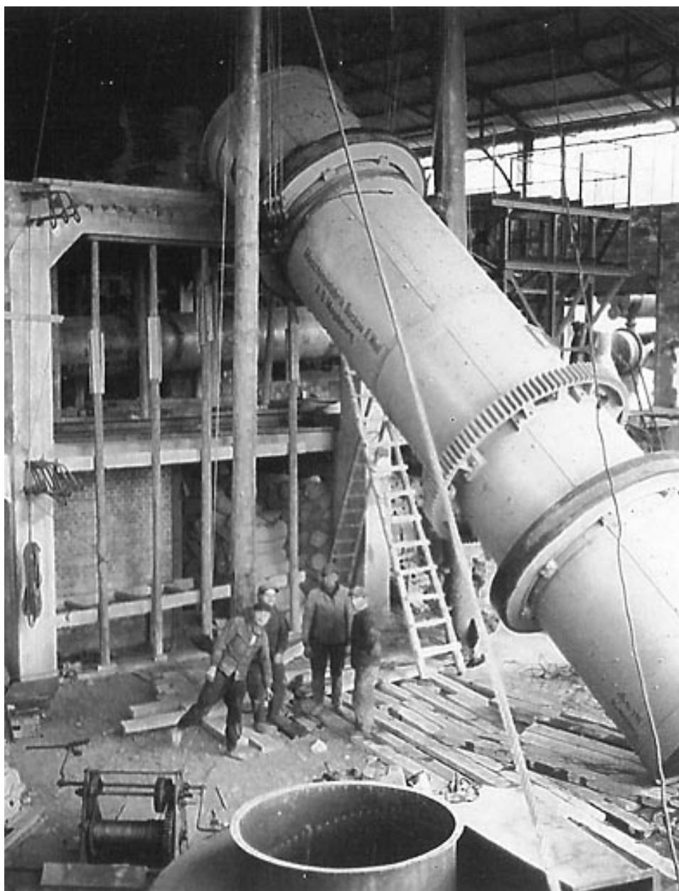
Mise en place du séchoir.
