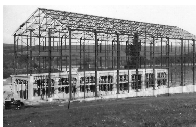
Raffinerie en cours de construction. Phot. Emile Hérissé, Phot. Emile Hérissé IVR43_20077000473NUCA
