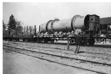
Le séchoir en gare de Creveney. Phot. Emile Hérissé, Phot. Emile Hérissé IVR43_20077000485NUCA
