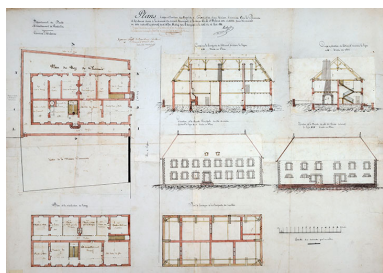
Plans, coupe et élévations du projet de construction d'une maison commune [...], 1832. Phot. Jérôme Mongreville
