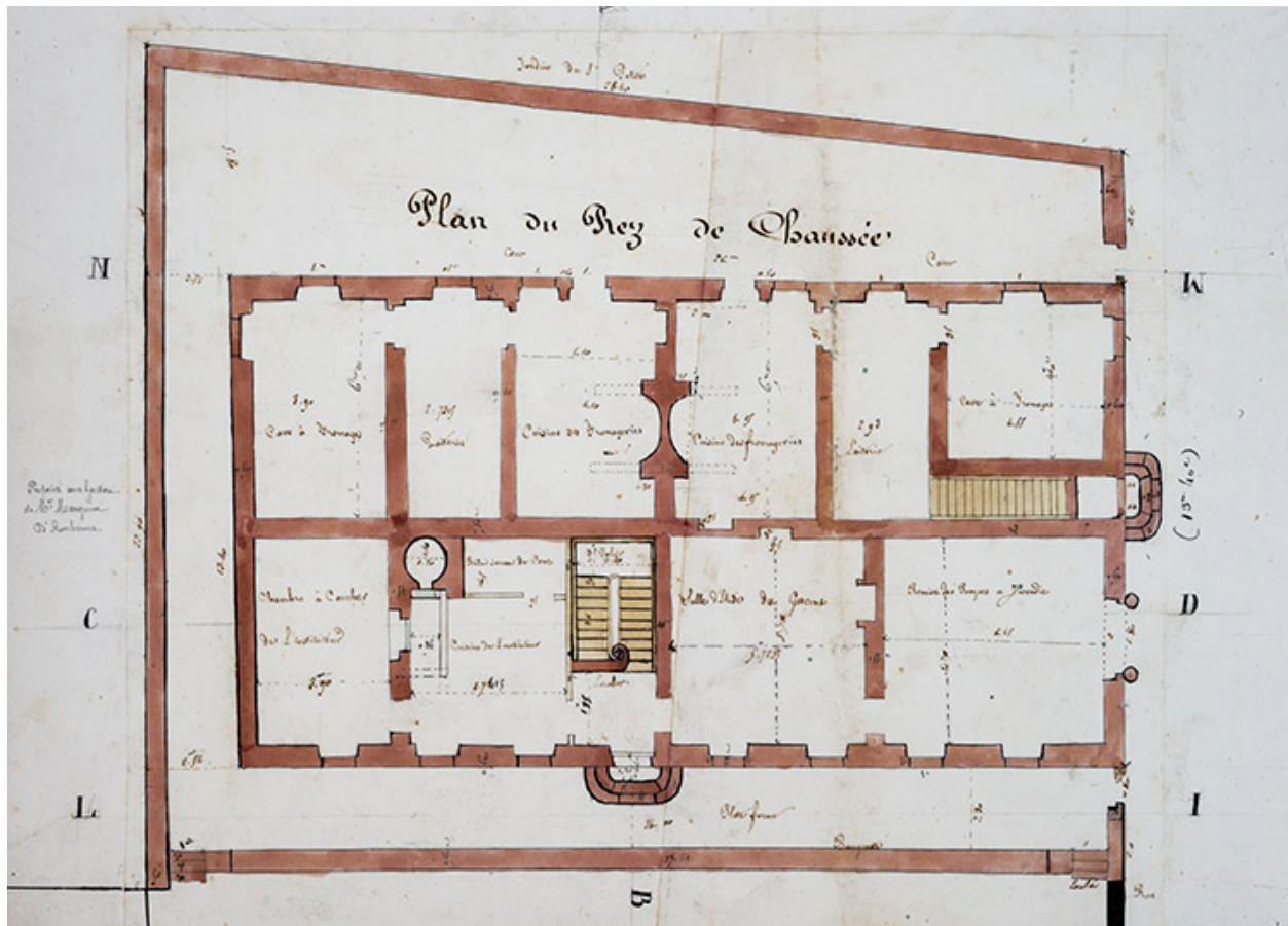
Plans, coupe et élévations du projet de construction d'une maison commune [...]. Plan du rez-de-chaussée, 1832.
