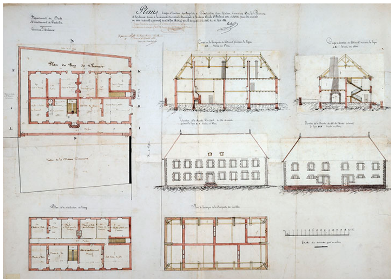
Plans, coupe et élévations du projet de construction d'une maison commune [...], 1832.
