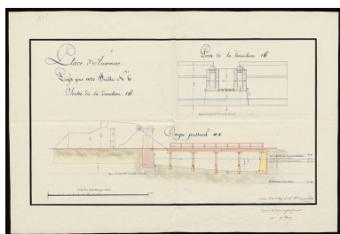
Projet pour 1820, coupe et élévation de la porte et du pont de la demi-lune 16. 1819. Autr. Piétit IVR26_20232100133NUC4A
