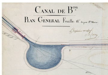
"Canal de Bourgogne. Plan général. Feuille 18e depuis Sainte-Marie". Souterrain et tranchée côté Escommes. 1811. (Archives départementales de la Côte-d'Or, Dijon) Phot. Thierry Kuntz, Autr. Charles Forey IVR26_20072100345NUC2A
