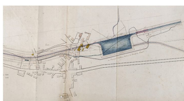
"Canal de Bourgogne. Plan général depuis Sainte-Marie". Souterrain et tranchée côté Pouilly. 1811. (Archives départementales de la Côte-d'Or, Dijon) Phot. Thierry Kuntz, Autr. Charles Forey IVR26_20072100346NUC2A
