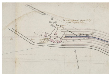
"Canal de Bourgogne. Plan général depuis Sainte-Marie". Souterrain et tranchée côté Pouilly. 1811. (Archives départementales de la Côte-d'Or, Dijon) Phot. Thierry Kuntz, Autr. Charles Forey IVR26_20072100344NUC2A
