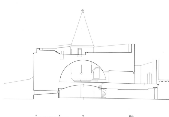
Boulevard dit Grosse Tour. Coupe B-B'. Dess. Alain Morelière IVR26_20122100982A2YY
