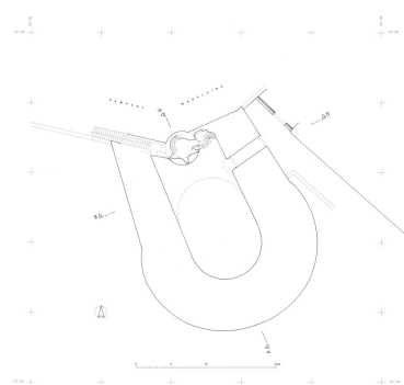
Boulevard dit Grosse Tour. Plan niveau supérieur. Dess. Alain Morelière IVR26_20122100073A1YY
