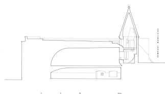
Boulevard dit Grosse Tour. Coupe A-A'. Dess. Alain Morelière IVR26_20122100981A2YY
