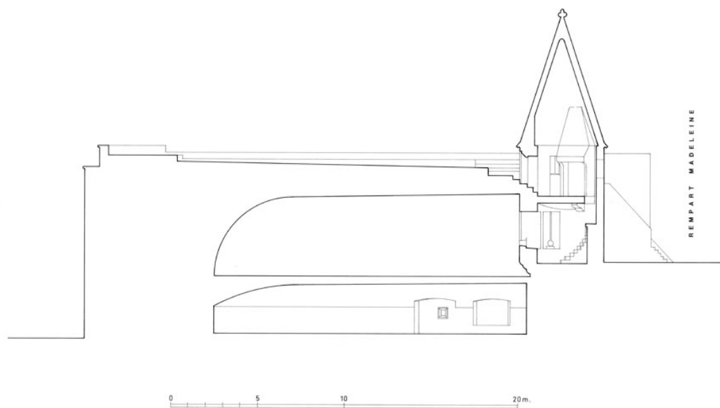
Boulevard dit Grosse Tour. Coupe A-A'.
