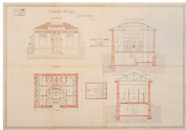
Bains douches, projet, 1906 [plan, coupes, élévation].
