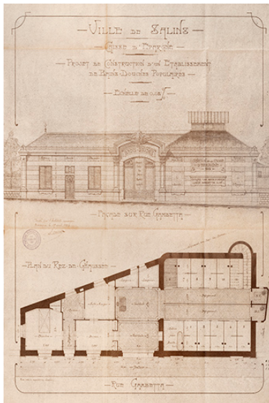
Ville de Salins - Caisse d'Epargne. Projet de construction d'un établissement de Bains douches populaires, 1913. Phot. Jérôme Mongreville IVR43_20233900878NUC4A
