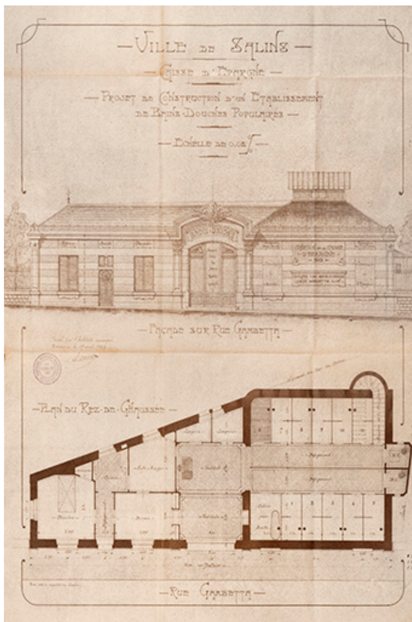
Ville de Salins - Caisse d'Epargne. Projet de construction d'un établissement de Bains douches populaires, 1913.
