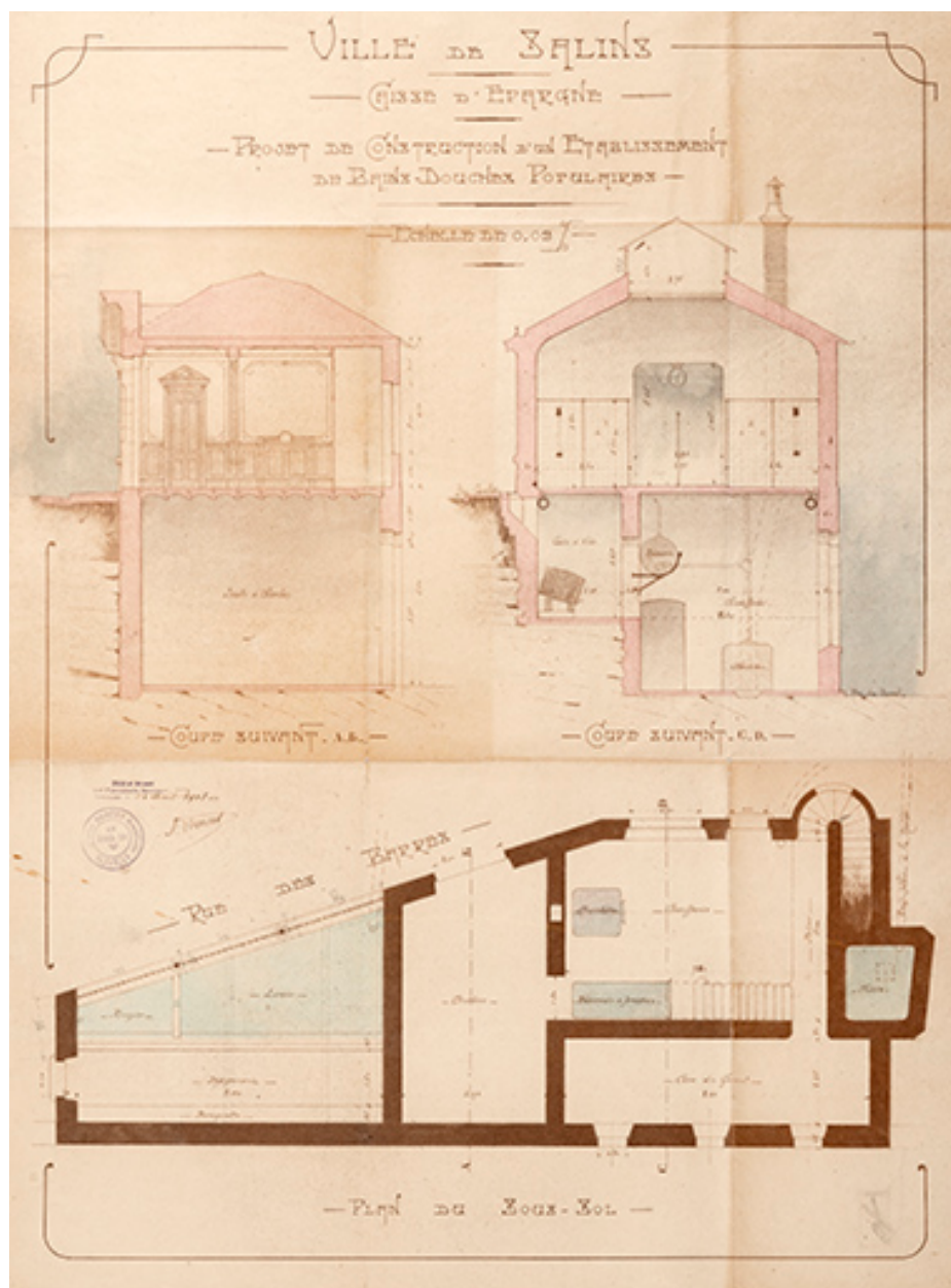
Ville de Salins - Caisse d'Epargne. Projet de construction d'un établissement de Bains douches populaires, 1913.
