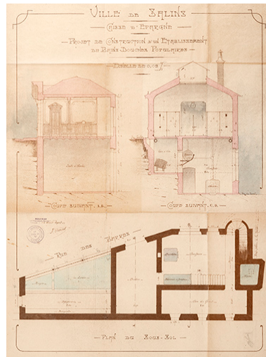
Ville de Salins - Caisse d'Epargne. Projet de construction d'un établissement de Bains douches populaires, 1913. Phot. Jérôme Mongreville IVR43_20233900879NUC4A
