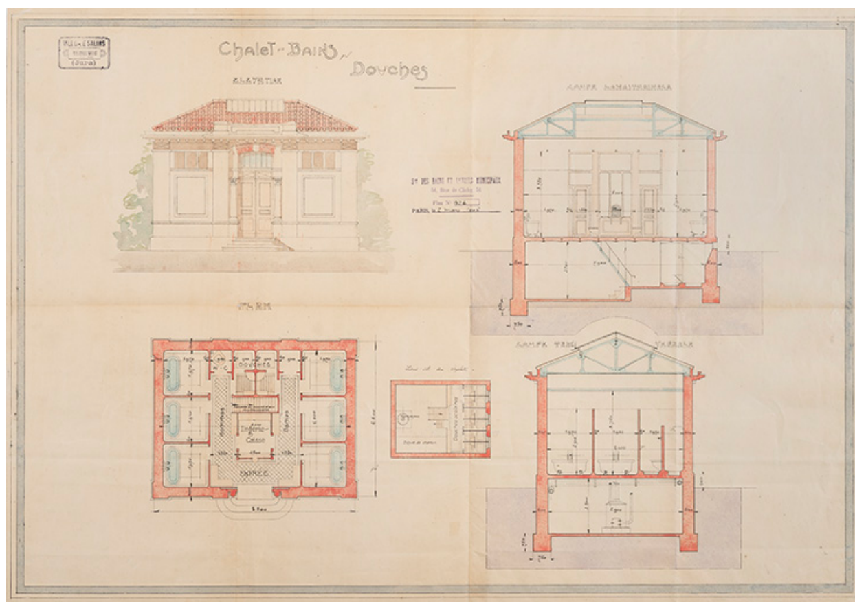
Bains douches, projet, 1906 [plan, coupes, élévation].
