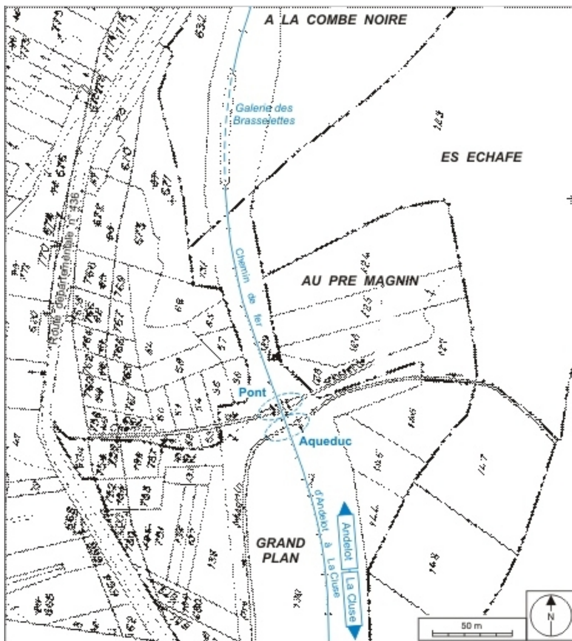
Plan-masse et de situation. Extrait du plan cadastral informatisé, 2006, section A, échelle 1:2500 agrandie à 1:2000.
