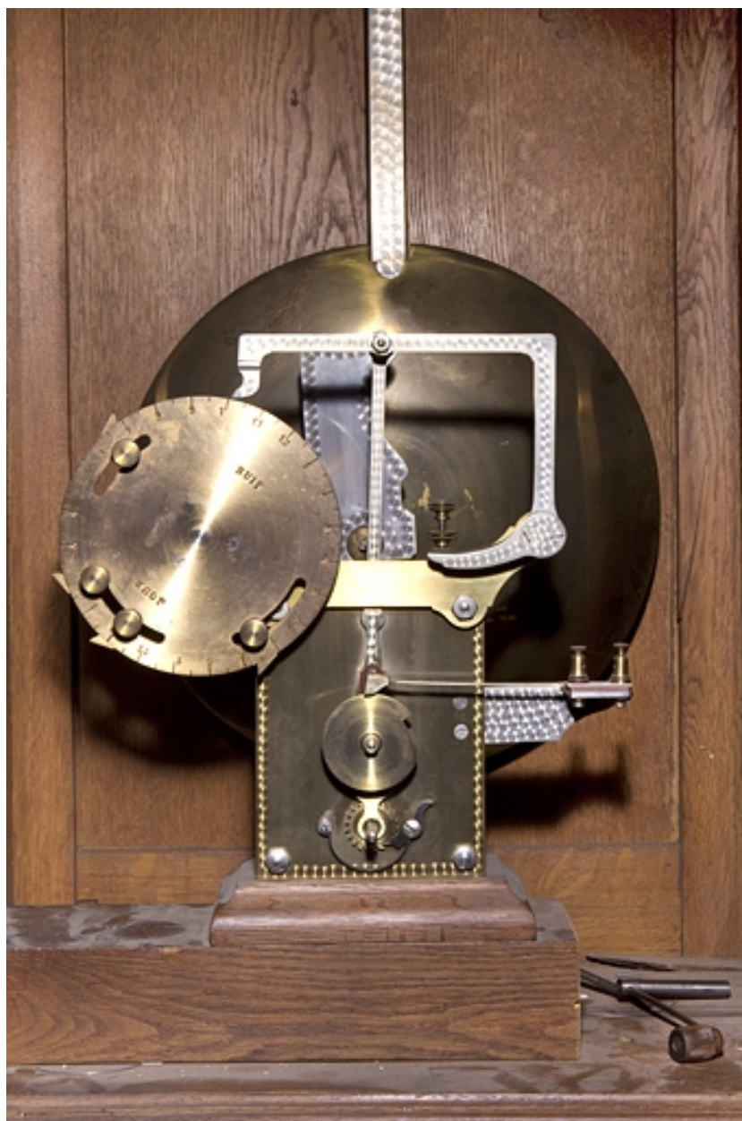
Système de programmation des sonneries.
