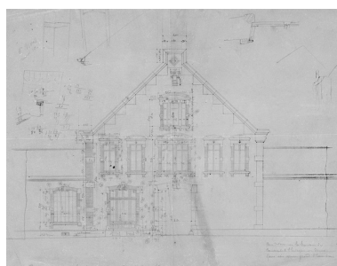
[Façade antérieure de la maison d'habitation de l'usine]. Phot. Jérôme Mongreville, Phot. Anthime Fleury de la Hussinière IVR43_20019000072V
