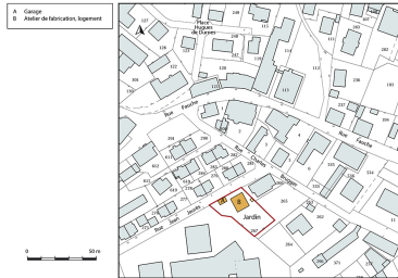
Plan-masse et de situation. Extrait du plan cadastral, 2018, section AA, 1/1 000. Dess. Bertrand Turina IVR43_20182501374NUDA
