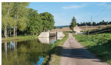
Vue du sas d'écluse depuis l'aval. Phot. Pierre-Marie Barbe-Richaud IVR26_20122101903NUC2AQ
