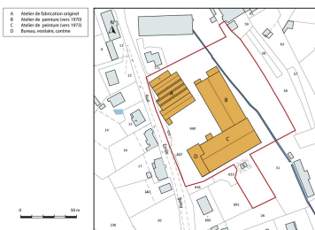
Plan-masse et de situation. Dess. Mathias Papigny IVR43_20132502589NUDA
