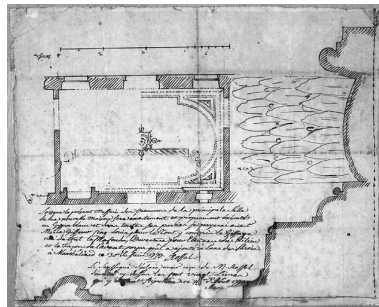
Plan du décor du plafond du grand salon, coupes des moulures, détail de la frise, 1773. Phot. Yves Sancey, Phot. Marca IVR43_19862500241V
