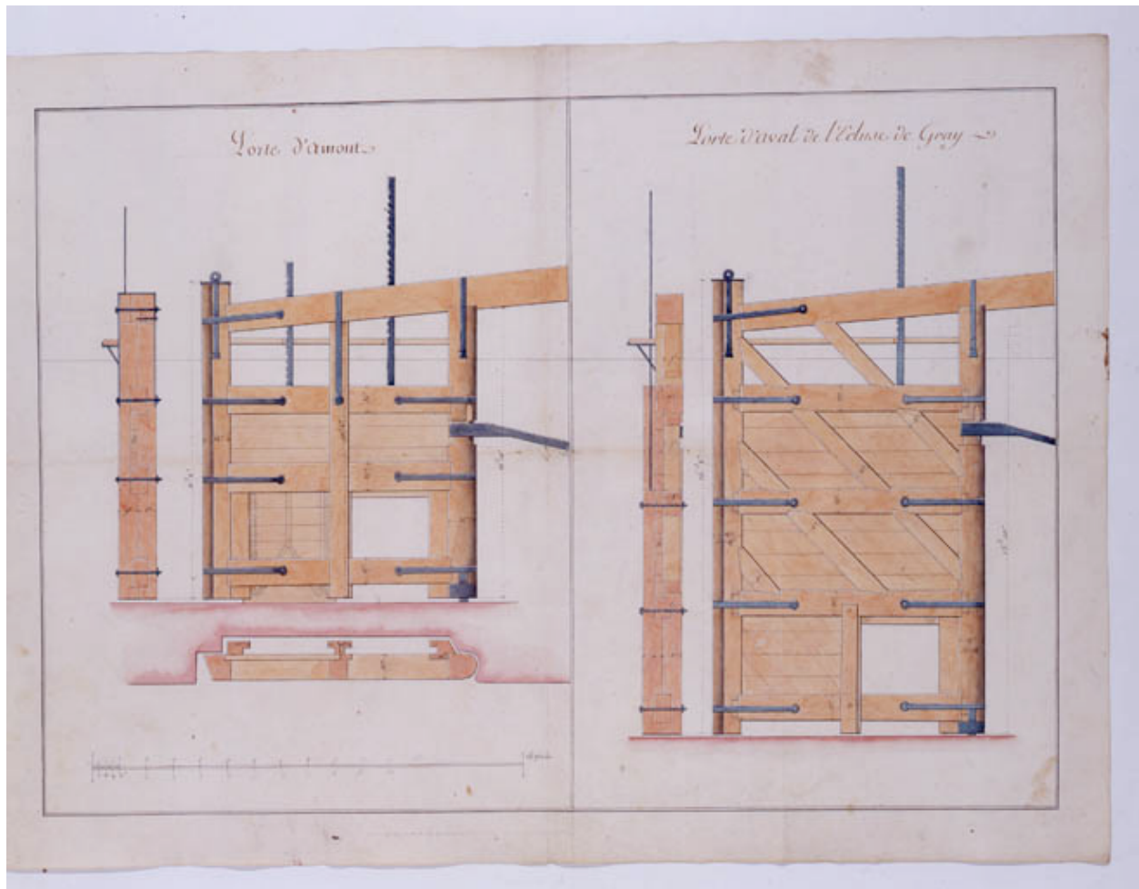
Portes d'amont et d'aval de l'écluse.
