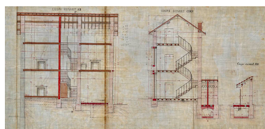
Achèvement du bief de Gray - Agrandissement de la maison éclusière, dessins d'exécution (1883). Phot. Jérôme Mongreville, Autr. Albert Hemardinquer IVR43_20207000198NUC4A
