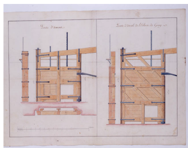
Portes d'amont et d'aval de l'écluse. Phot. Yves Sancey, Autr. Philippe Bertrand IVR43_19927000278VA
