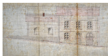
Achèvement du bief de Gray - Agrandissement de la maison éclusière, dessins d'exécution (1883). Phot. Jérôme Mongreville, Autr. Albert Hemardinquer IVR43_20207000196NUC4A
