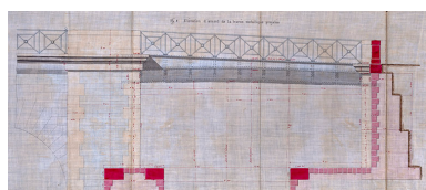
Construction de la partie métallique de la travée marinière du pont de Gray - Plan, élévation, coupes et détails (1882). Phot. Jérôme Mongreville, Autr. Gustave Bouvaist IVR43_20207000200NUC4A
