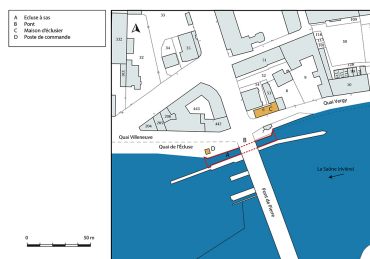
Plan masse et de situation. Dess. Bertrand Turina IVR43_20207000773NUDA
