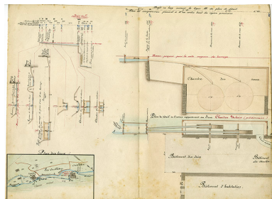
Ruisseau de Derrière-le-Mont. Commune de Montlebon. Règlement d'eau de l'usine du sieur Chardon Urbain. Plan, profils en long et en travers et dessins de détails, 1863. Autr. Cuvinot IVR43_20182500035NUC4A
