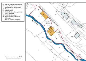
Plan-masse et de situation. Extrait du plan cadastral, 2016, section D, 1/1 000. Dess. Bertrand Turina IVR43_20182501333NUDA
