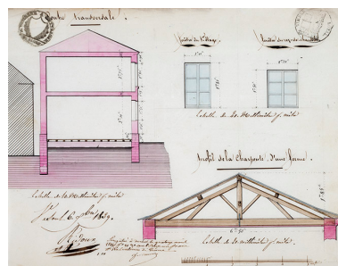
Plan en coupe de la maison commune et détails des fenêtres et de la charpente, 1839 Phot. Jérôme Mongreville, Autr. Jean-Baptiste Ridoux IVR43_20167001583NUC4A
