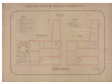
Plans de l'école des filles et logements des instituteurs Phot. Jérôme Mongreville IVR43_20167001513NUC2A
