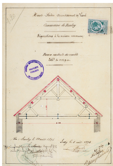
Réparations à la maison commune, plan en coupe de la ferme centrale du comble, 1894 Phot. Jérôme Mongreville, Autr. J.-B. Martin IVR43_20167001588NUC4A
