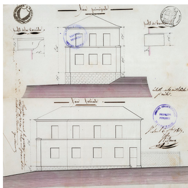
Plans en élévation des façades de la maison commune, 1839 Phot. Jérôme Mongreville, Autr. Jean-Baptiste Ridoux IVR43_20167001584NUC4A
