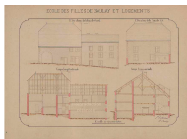
Plans de l'école des filles et logements des instituteurs Phot. Jérôme Mongreville IVR43_20167001512NUC2A
