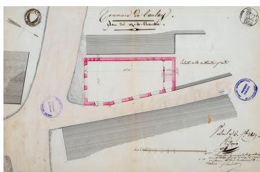
Plan en coupe du rez-de-chaussée de la maison commune, 1839 Phot. Jérôme Mongreville, Autr. Jean-Baptiste Ridoux IVR43_20167001587NUC4A
