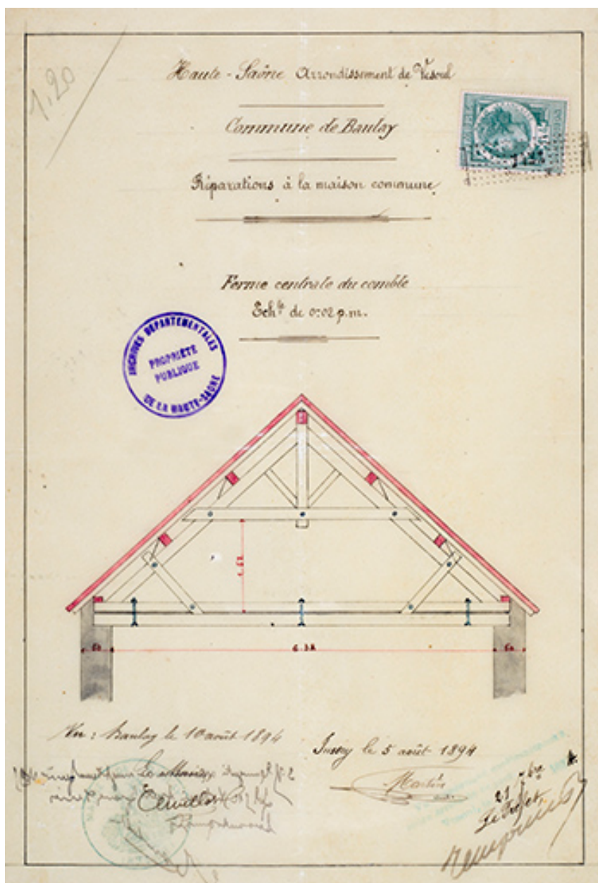
Réparations à la maison commune, plan en coupe de la ferme centrale du comble, 1894
