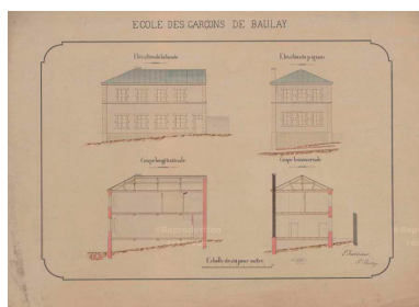
Plans de l'école des garçons Phot. Jérôme Mongreville IVR43_20167001510NUC2A
