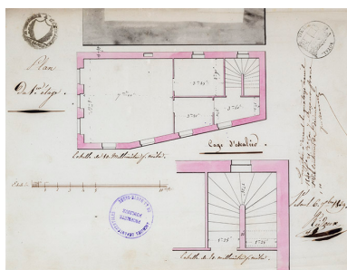
Plan en coupe du premier étage de la maison commune, 1839 Phot. Jérôme Mongreville, Autr. Jean-Baptiste Ridoux IVR43_20167001586NUC4A
