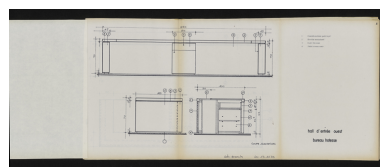
Carnet de détails et principes - hall d'entrée ouest : bureau des hôtesse, coupe et élévations, 13 novembre 1978. Boyer, Michel (architecte d'intérieur) (Archives départementales de la Côte-d'Or, Dijon, 32 J 106) Phot. Petot Frédéric, Autr. Michel (architecte d'intérieur) Boyer IVR26_20142100796NUC2A
