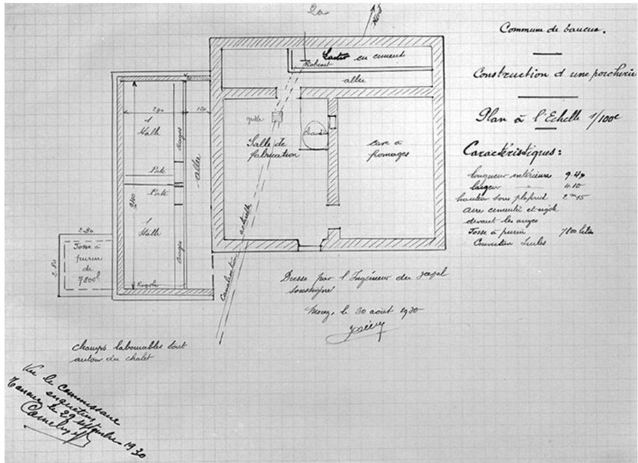
Construction d'une porcherie : plan du rez-de-chaussée, 1930.
