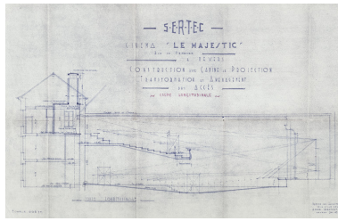
SERTEC Cinéma 'Le Majestic' rue de Nemours à Nevers. Construction d'une cabine de projection [...] Coupe longitudinale. Décembre 1947.
