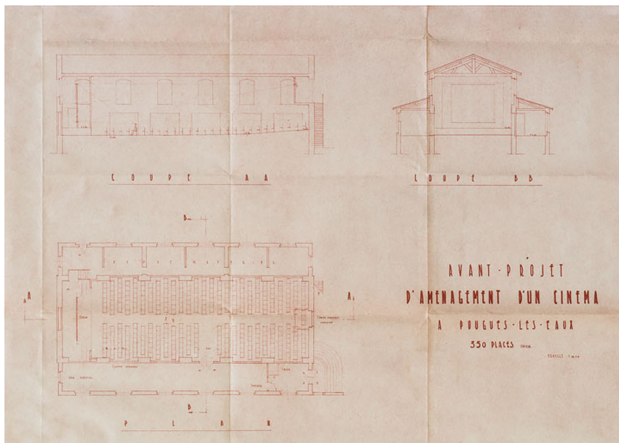
Avant-projet d'aménagement d'un cinéma à Pougues-les-Eaux. 350 places environ. 1950.
