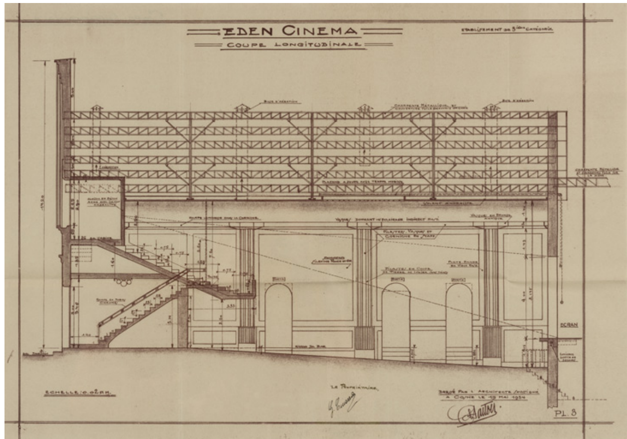
Eden-Cinéma [à Cosne-Cour-sur-Loire. Plans, coupes et élévation]. 1934.
