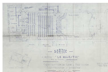
SERTEC Cinéma 'Le Majestic' rue de Nemours à Nevers. Construction d'une cabine de projection [...] Plan au niveau du balcon et de la cabine. Décembre 1947. Phot. Pierre-Marie Barbe-Richaud, Autr. Roger Rouvet IVR26_20245800786NUC4A
