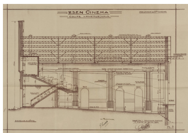
Eden-Cinéma [à Cosne-Cour-sur-Loire. Plans, coupes et élévation]. 1934. Phot. Pierre-Marie Barbe-Richaud, Autr. Roger Charton IVR26_20245800292NUC4A
