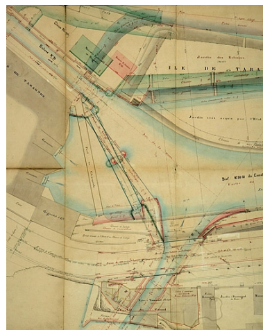
Dérivation sous la citadelle de Besançon. Plan des ouvrages à l'extrémité aval de la dérivation, 1877. Phot. Yves Sancey, Phot. Rascol IVR43_20062500092NUCA
