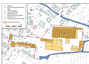
Plan-masse et de situation. Dess. Mathias Papigny IVR43_20132502572NUDA
