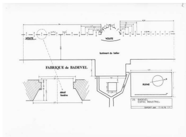
Plan-masse de l'atelier d'horlogerie en 1981.
