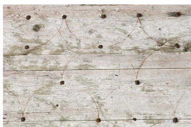
Ferme d'Entre-les-Fourgs (rue de Jougne, 2020 AD 173 ?) : détail d'une porte de grange montrant les tracés au compas utilisés pour positionner les clous de manière régulière.
