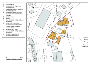
Plan-masse et de situation. Extrait du plan cadastral, 2018, Les Fins section AK et Morteau section AD, 1/1 000. Dess. Bertrand Turina IVR43_20182501402NUDA
