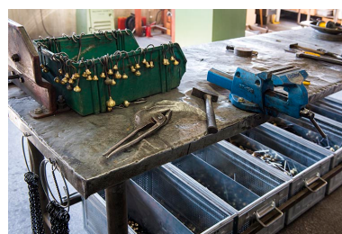
Etabli pour le montage des battants (vue rapprochée). Phot. Sonia Dourlot IVR43_20182501095NUC4A
