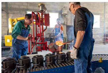
Coulée dans un petit châssis. Phot. Sonia Dourlot IVR43_20182501058NUC4A
