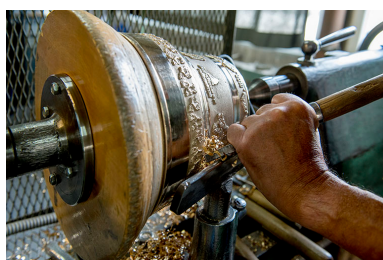
Tournage d'une cloche : position du ciseau. Phot. Sonia Dourlot IVR43_20182501092NUC4A
