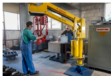
Fonte du bronze (la grue est prête à saisir la poche de métal en fusion). Phot. Sonia Dourlot IVR43_20182501056NUC4A
