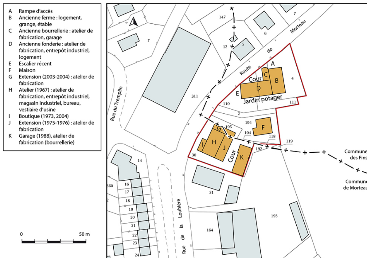
Plan-masse et de situation. Extrait du plan cadastral, 2018, Les Fins section AK et Morteau section AD, 1/1 000.
