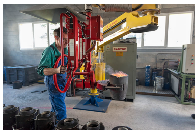
Transport du creuset (poche) plein de bronze en fusion, à l'aide de la grue d'atelier. Phot. Sonia Dourlot IVR43_20182501057NUC4A
