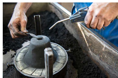
Fabrication du moule : finition du moulage en relief (intérieur de la cloche) une fois le modèle retiré.
