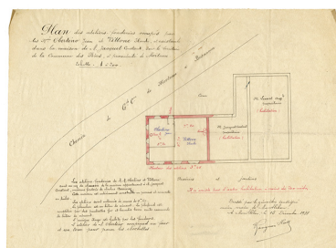
Plan des ateliers-fonderies occupés par les [nommés] Obertino Jean et Vittone Ilardo [...], 15 décembre 1931. Phot. Sonia Dourlot, Autr. Rougnon-Glasson IVR43_20192500896NUC2A
