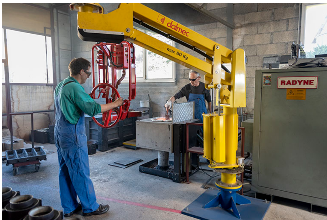
Fonte du bronze (la grue est prête à saisir la poche de métal en fusion).
