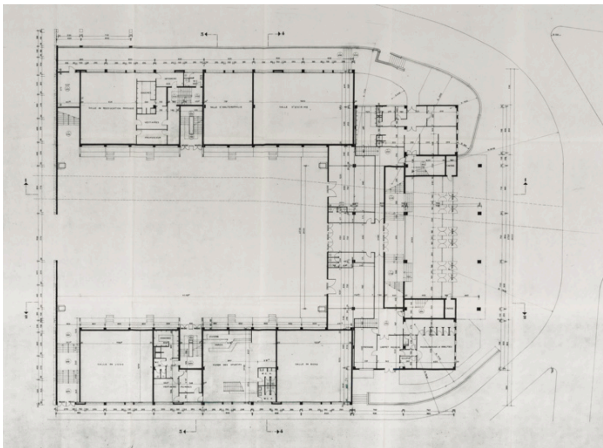
Nevers Centre municipal. Maison des sports. 5. Plan d'exécution. Niveaux -350 -600. Octobre 1964.
