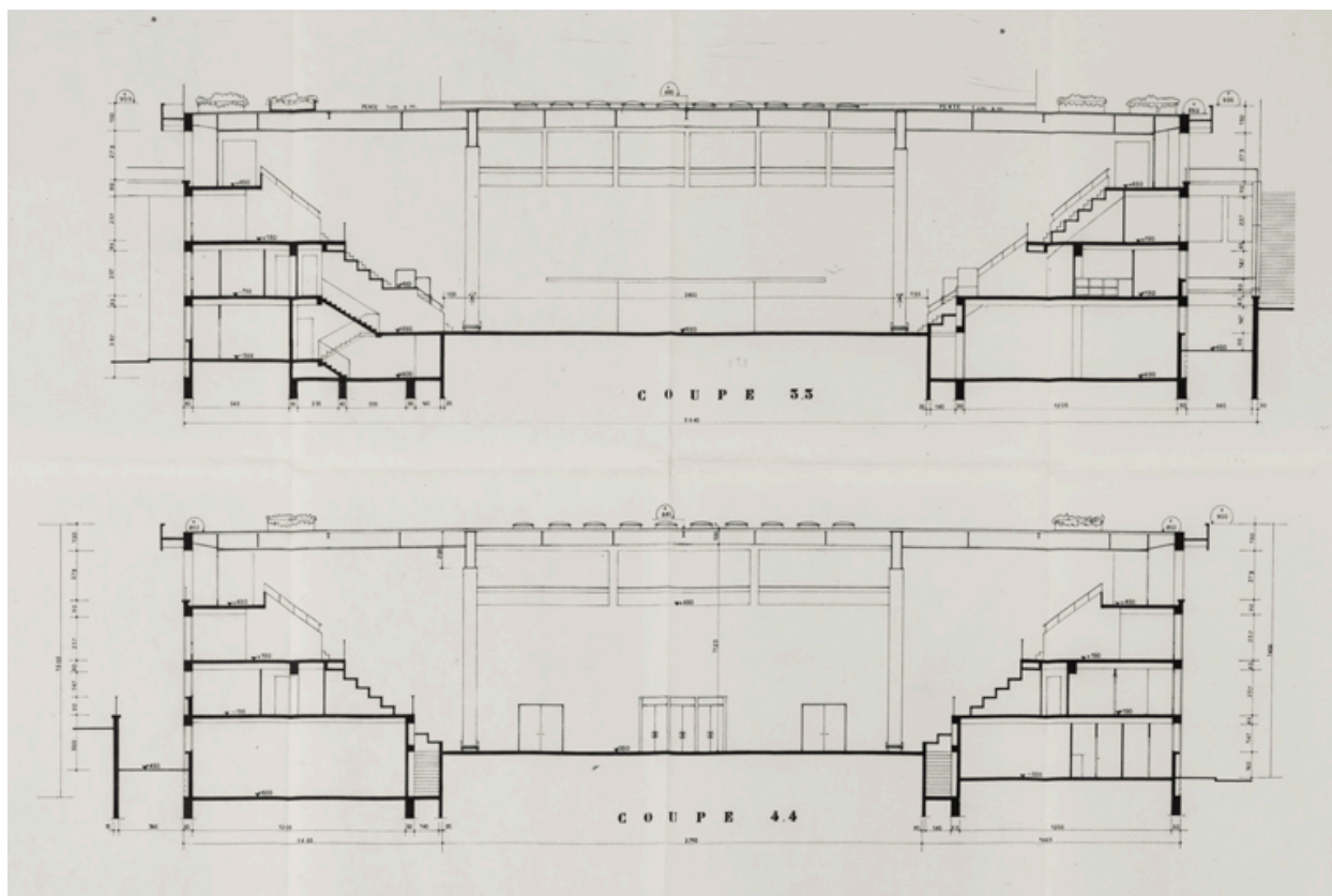
Nevers Centre municipal. Maison des sports. 10. Plan d'exécution. Coupes transversales. Octobre 1964.
