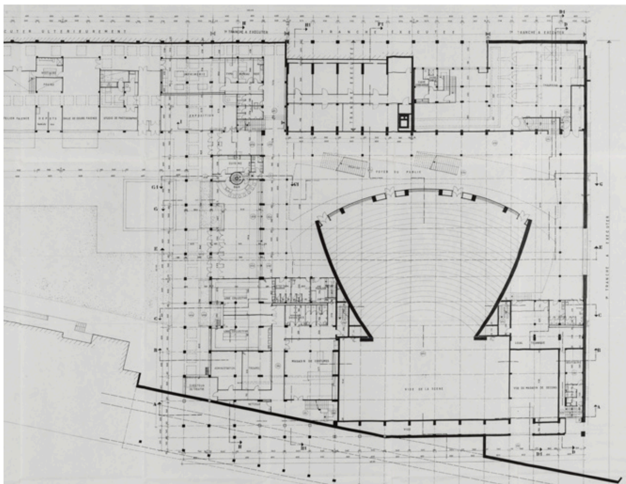
Nevers Centre municipal. Maison de la culture. 6. Plan d'exécution. Niveau jardin, parterre théâtre [... Détail : partie droite]. Octobre 1964, rect. novembre 1964.
