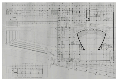
Nevers Centre municipal. Maison de la culture. 7. Plan d'exécution.
