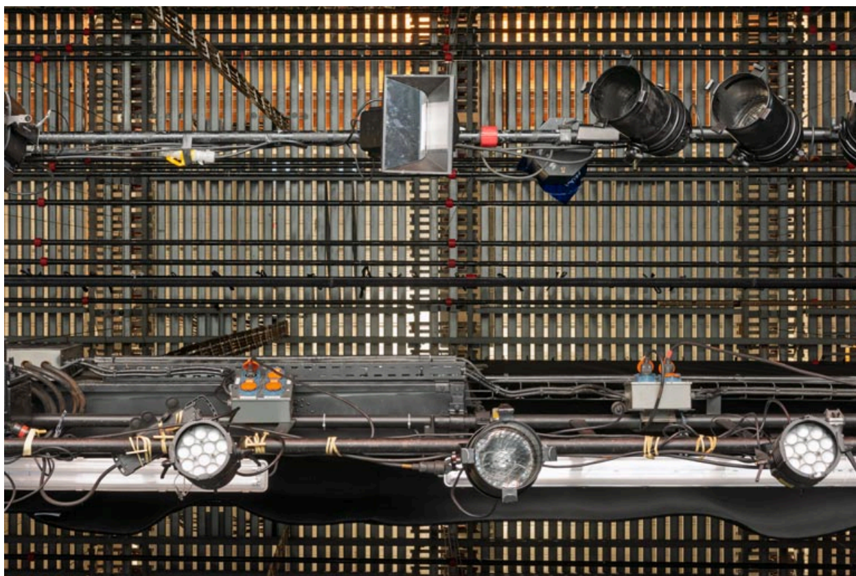
Maison de la culture, grande salle : le gril, vu de la scène, et perches portant des projecteurs.
