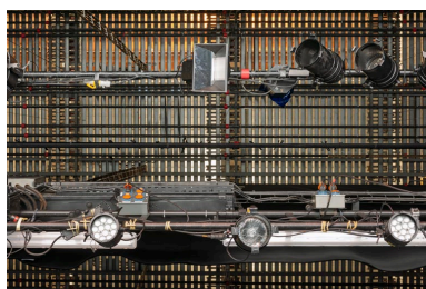
Maison de la culture, grande salle : le gril, vu de la scène, et perches portant des projecteurs. Phot. Pierre-Marie Barbe-Richaud IVR26_20245800922NUC4A
