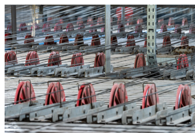
Maison de la culture, grande salle : poulies sur le le gril. Phot. Pierre-Marie Barbe-Richaud IVR26_20245800949NUC4A
