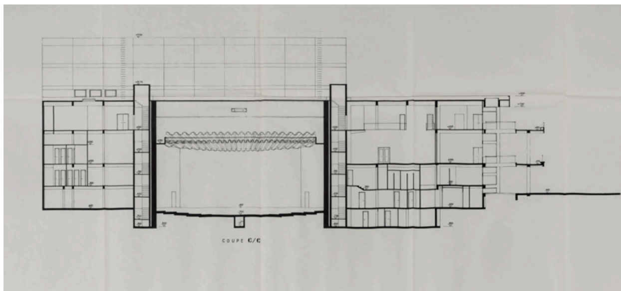
Nevers Centre municipal. Maison de la culture. 11. Plan d'exécution. Coupe transversale sur la salle C/C. Octobre 1964.
