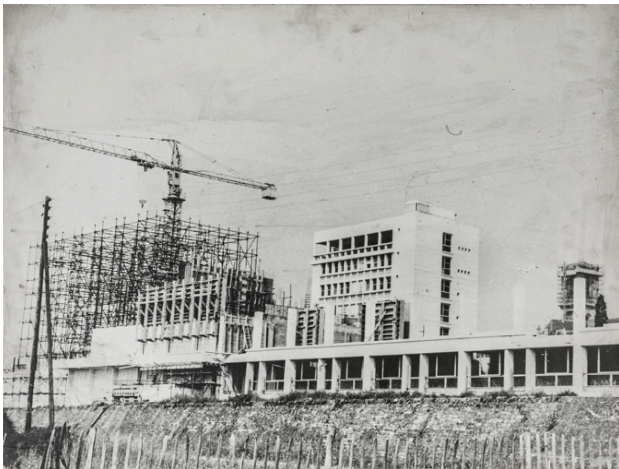
[Maison de la culture et des sports. Construction de la cage de scène]. S.d. [1967-1968].
