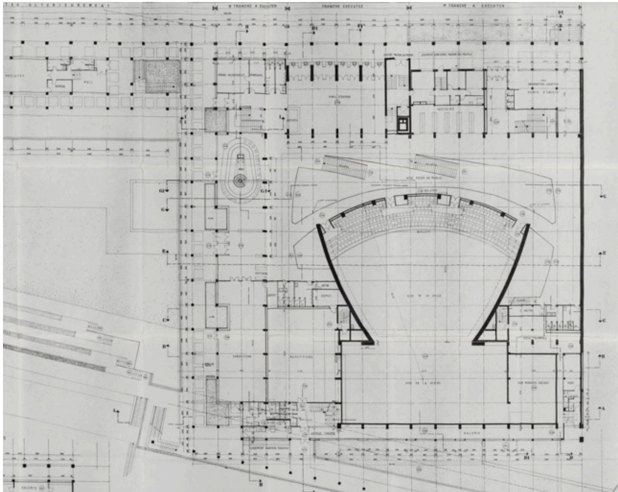
Nevers Centre municipal. Maison de la culture. 7. Plan d'exécution. Niveau rue, hall d'entrée [... Détail : partie droite]. Octobre 1964, rect. novembre 1964.
