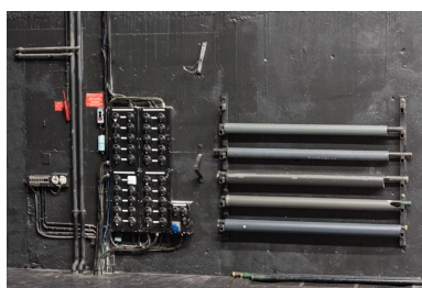
Maison de la culture, grande salle : boîtiers d'alimentation, au lointain sur la scène. Phot. Pierre-Marie Barbe-Richaud IVR26_20245800924NUC4A
