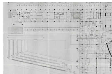
Nevers Centre municipal. Maison de la culture. 6. Plan d'exécution. Niveau jardin, parterre théâtre [... Détail : partie gauche]. Octobre 1964, rect. novembre 1964. Phot. Pierre-Marie Barbe-Richaud, Autr. Max Guillaume, Autr. Henri Vauzelle IVR26_20245800815NUC4A
