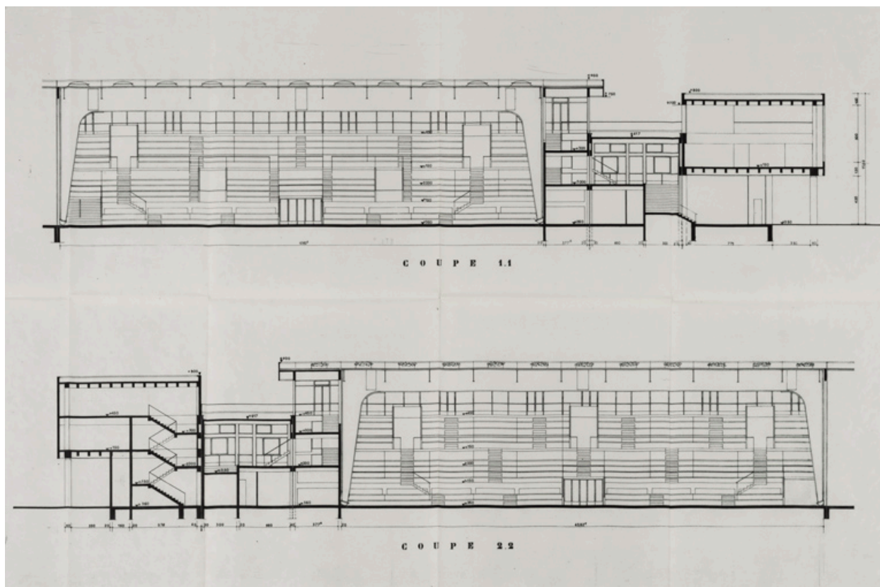
Nevers Centre municipal. Maison des sports. 11. Plan d'exécution. Coupes longitudinales. Octobre 1964.
