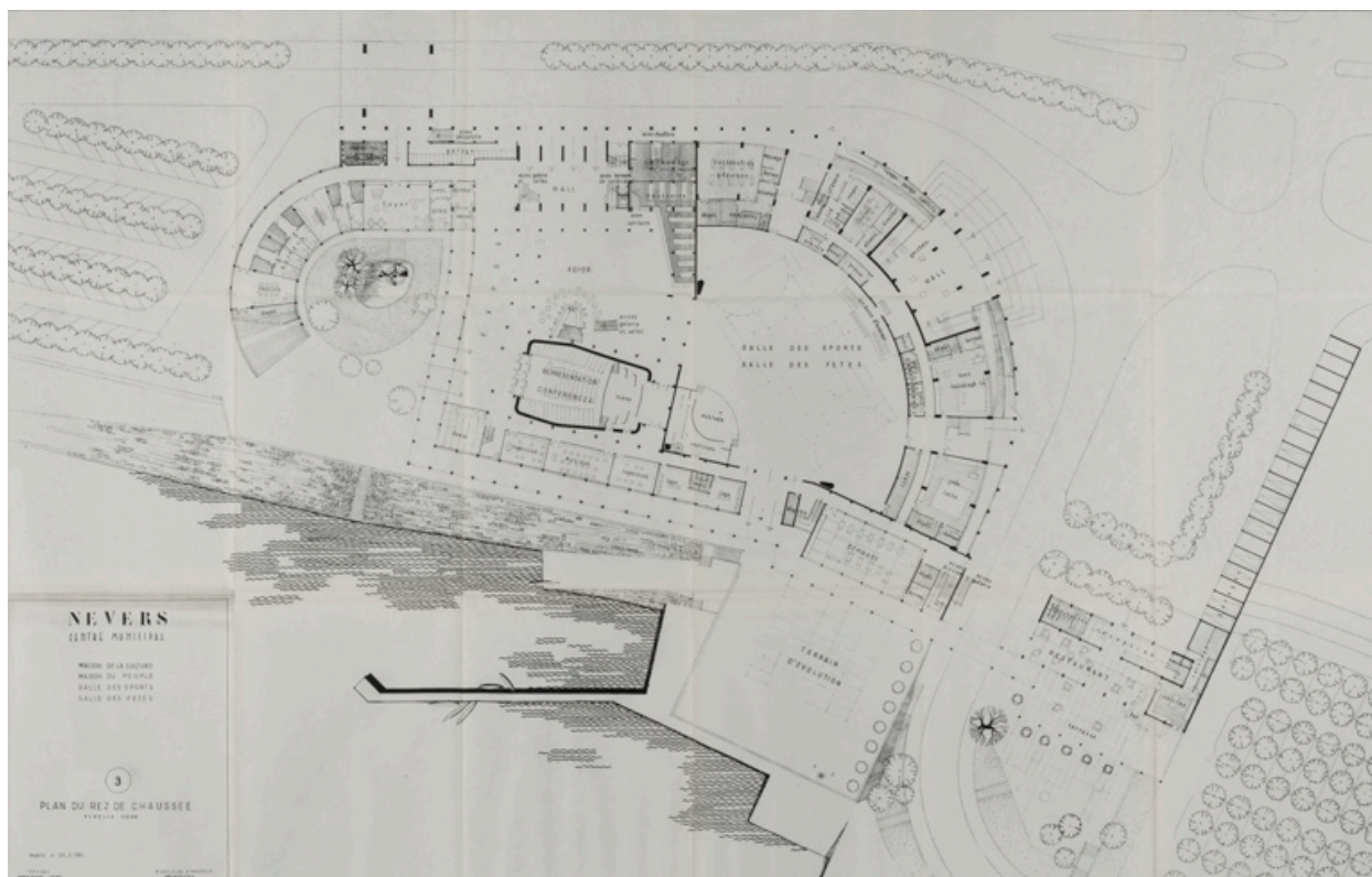
Nevers Centre municipal [...] 3. Plan du rez de chaussée. Novembre 1960-mars 1961.
