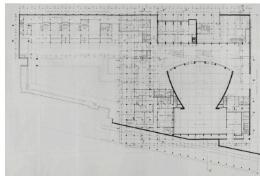
Nevers Centre municipal. Maison de la culture. 6. Plan d'exécution. Niveau jardin, parterre théâtre, loges collectives, ateliers artistes -150 -300 -350 -400. Octobre 1964, rect. novembre 1964. Phot. Pierre-Marie Barbe-Richaud, Autr. Max Guillaume, Autr. Henri Vauzelle IVR26_20245800817NUC4A
