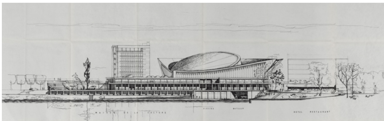
Nevers Centre municipal [...] 8. Façade sur Loire - S. E. Novembre 1960-mars 1961.
