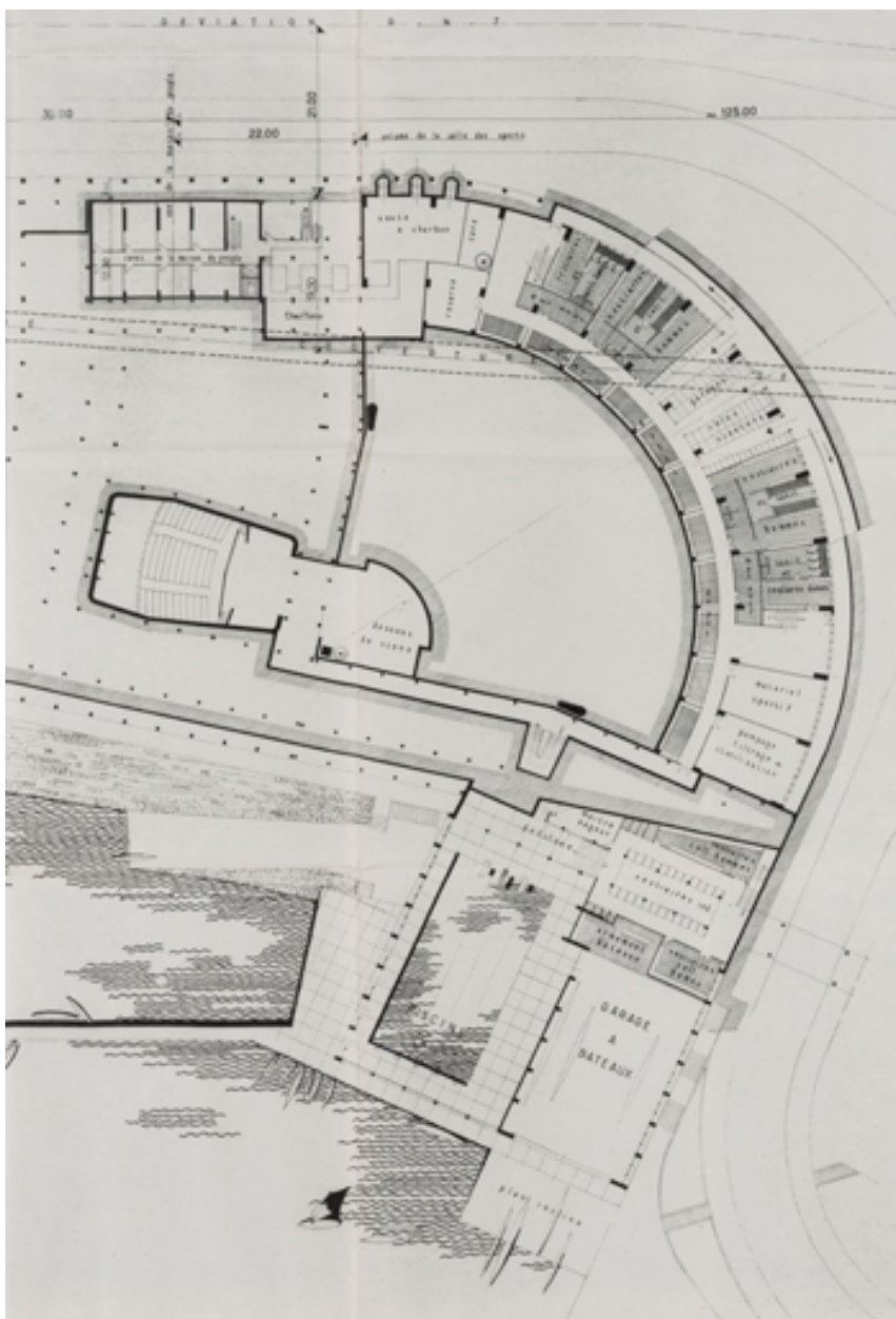
Nevers Centre municipal [...] 2B. Plan de sous-sol [détail]. Novembre 1960-mars 1961.
