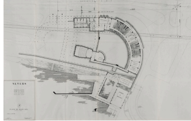
Nevers Centre municipal [...] 2B. Plan de sous-sol. Novembre 1960-mars 1961. Phot. Pierre-Marie Barbe- Richaud, Autr. Max Guillaume, Autr. Henri Vauzelle IVR26_20245800790NUC4A
