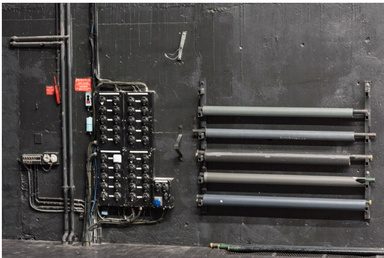
Maison de la culture, grande salle : boîtiers d'alimentation, au lointain sur la scène.
