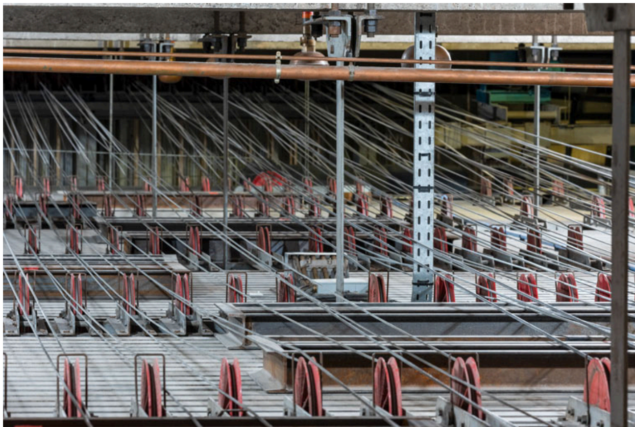
Maison de la culture, grande salle : le gril, vue rapprochée de trois quarts.
