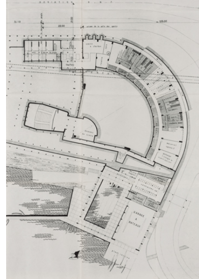
Nevers Centre municipal [...] 2B. Plan de sous-sol [détail]. Novembre 1960-mars 1961. Phot. Pierre-Marie Barbe- Richaud, Autr. Max Guillaume, Autr. Henri Vauzelle IVR26_20245800789NUC4A
