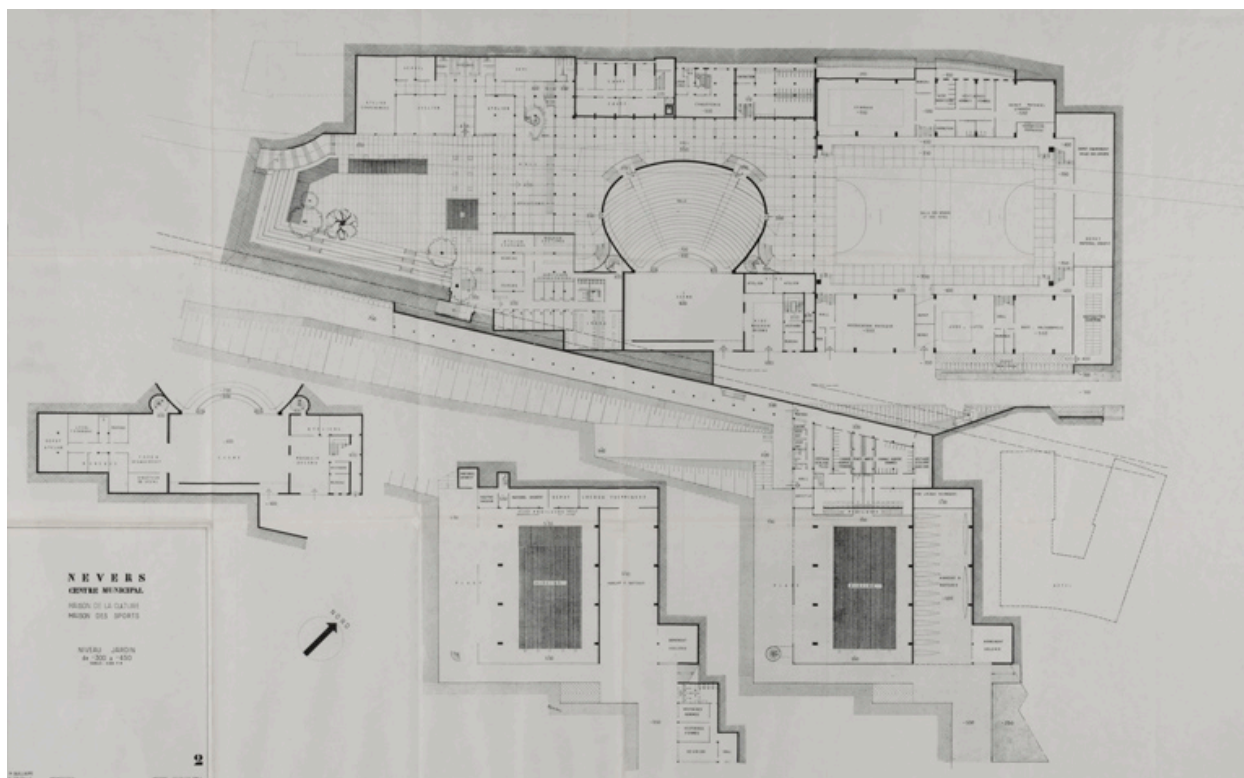
Nevers Centre municipal. Maison de la culture, maison des sports. 2. Niveau jardin de -300 à -450. Février 1963.
