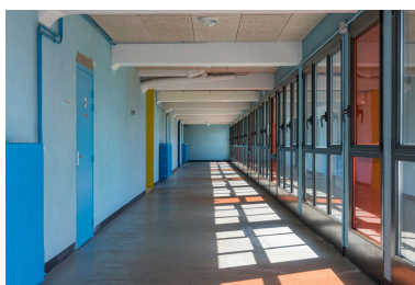
Maison des sports, grand gymnase : galerie vitrée à mi-hauteur des gradins côté Loire. Phot. Pierre-Marie Barbe-Richaud IVR26_20245800883NUC4A
