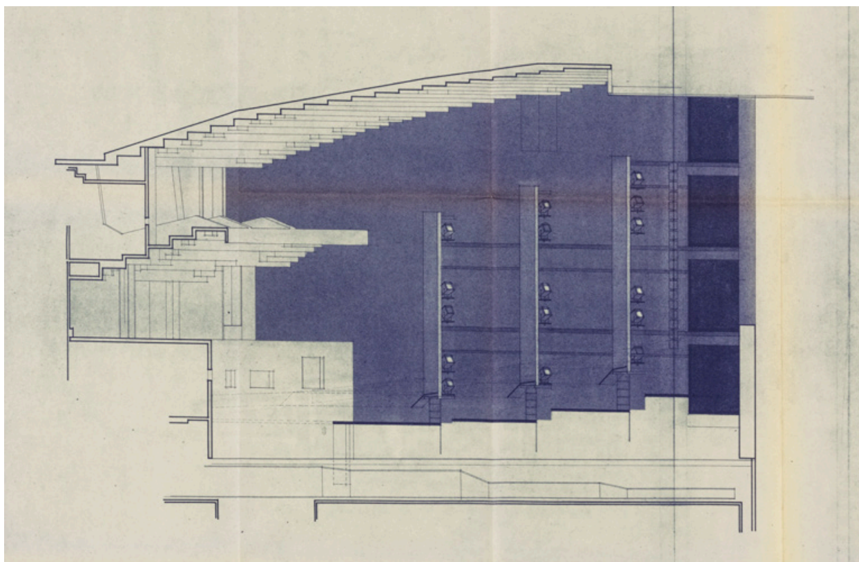
Ville de Nevers. Maison de la culture. Equipement scénique.SC 18. Plan du plafond de la salle et parois latérales [détail : parois]. 1968.
