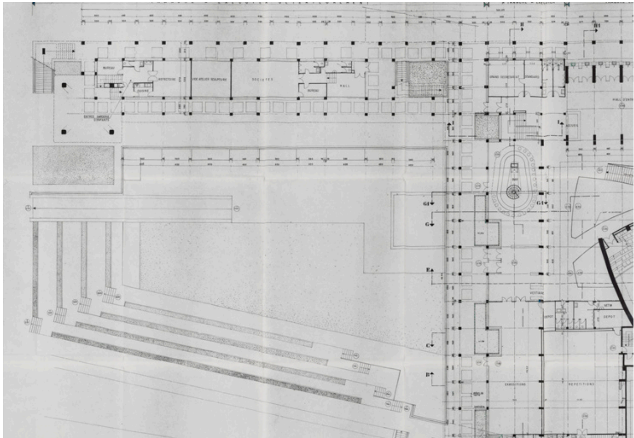
Nevers Centre municipal. Maison de la culture. 7. Plan d'exécution. Niveau rue, hall d'entrée [... Détail : partie gauche]. Octobre 1964, rect. novembre 1964.
