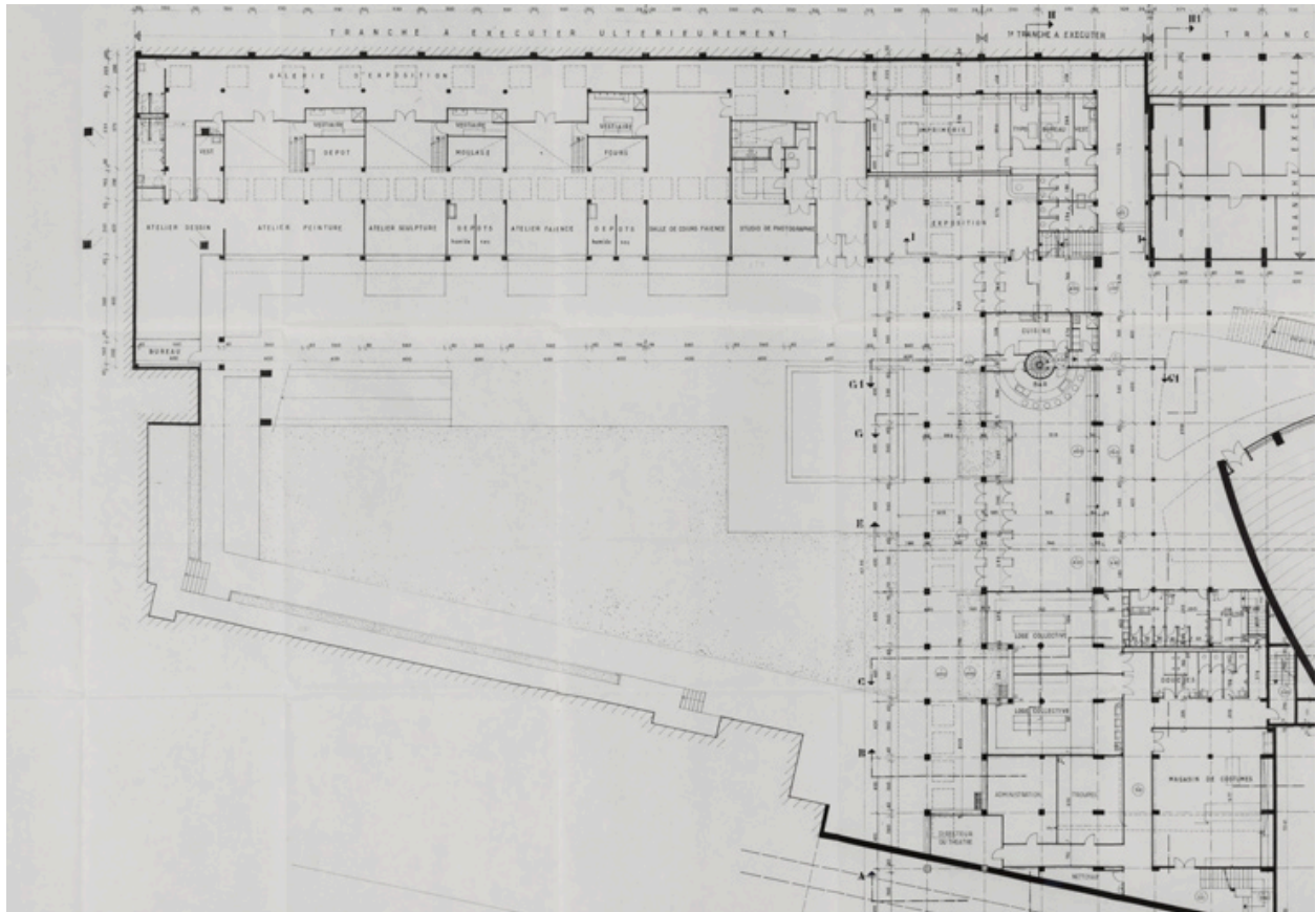
Nevers Centre municipal. Maison de la culture. 6. Plan d'exécution. Niveau jardin, parterre théâtre [... Détail : partie gauche]. Octobre 1964, rect. novembre 1964.
