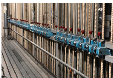
Maison de la culture, grande salle : freins à levier des équipes contrebalancées, sur la passerelle de commande (vue rapprochée). Phot. Pierre-Marie Barbe-Richaud IVR26_20245800939NUC4A
