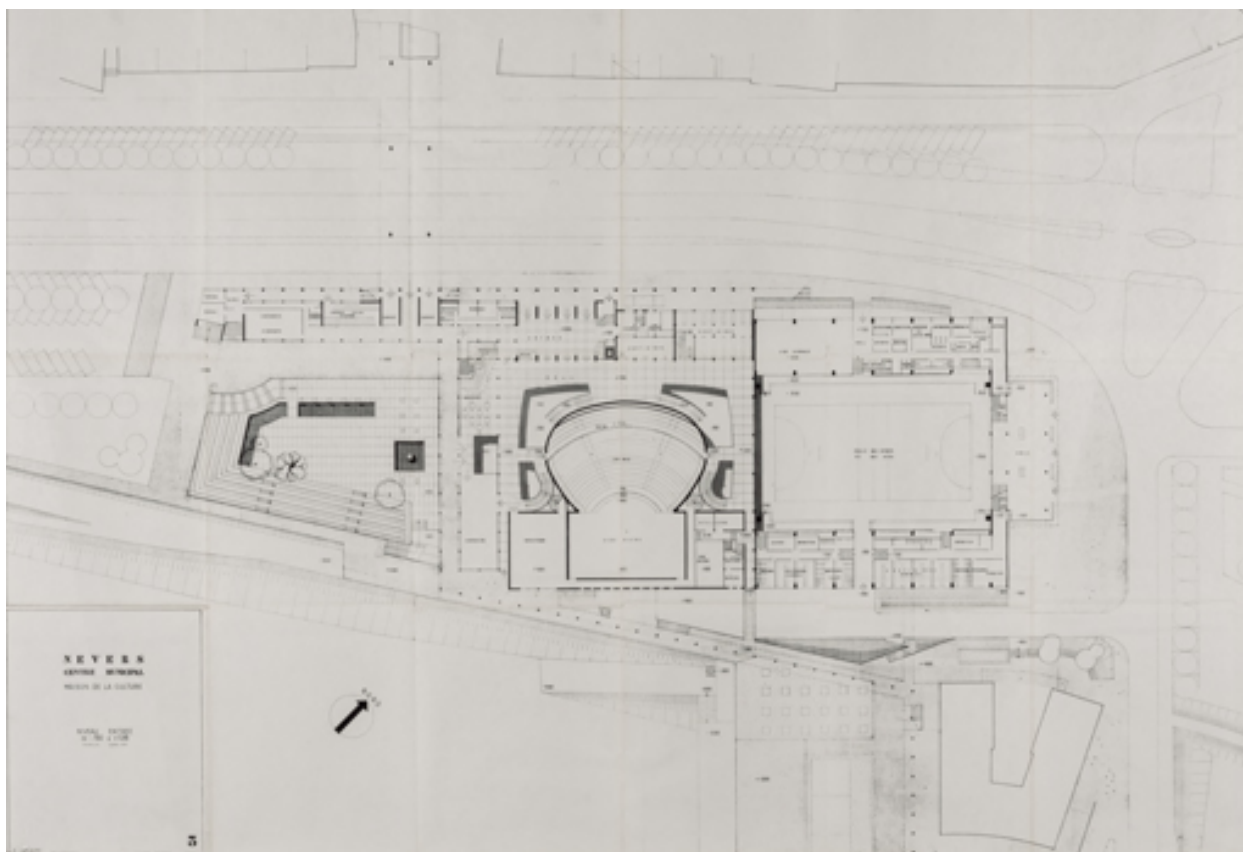
Nevers Centre municipal. Maison de la culture, maison des sports. 3. Niveau entrée de -150 à +128. Février 1963.
