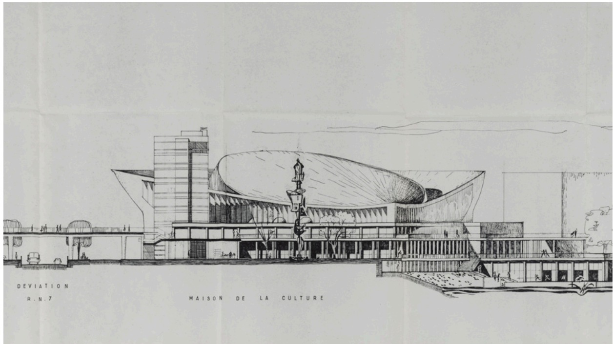
Nevers Centre municipal [...] 9. Façade sur maison de la culture - S. O. [détail]. Novembre 1960-mars 1961.
