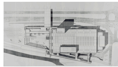
Nevers Centre municipal. Maison de la culture. 1. Plan d'ensemble [détail]. Octobre 1964, rect. novembre 1964. Phot. Pierre-Marie Barbe-Richaud, Autr. Max Guillaume, Autr. Henri Vauzelle IVR26_20245800811NUC4A
