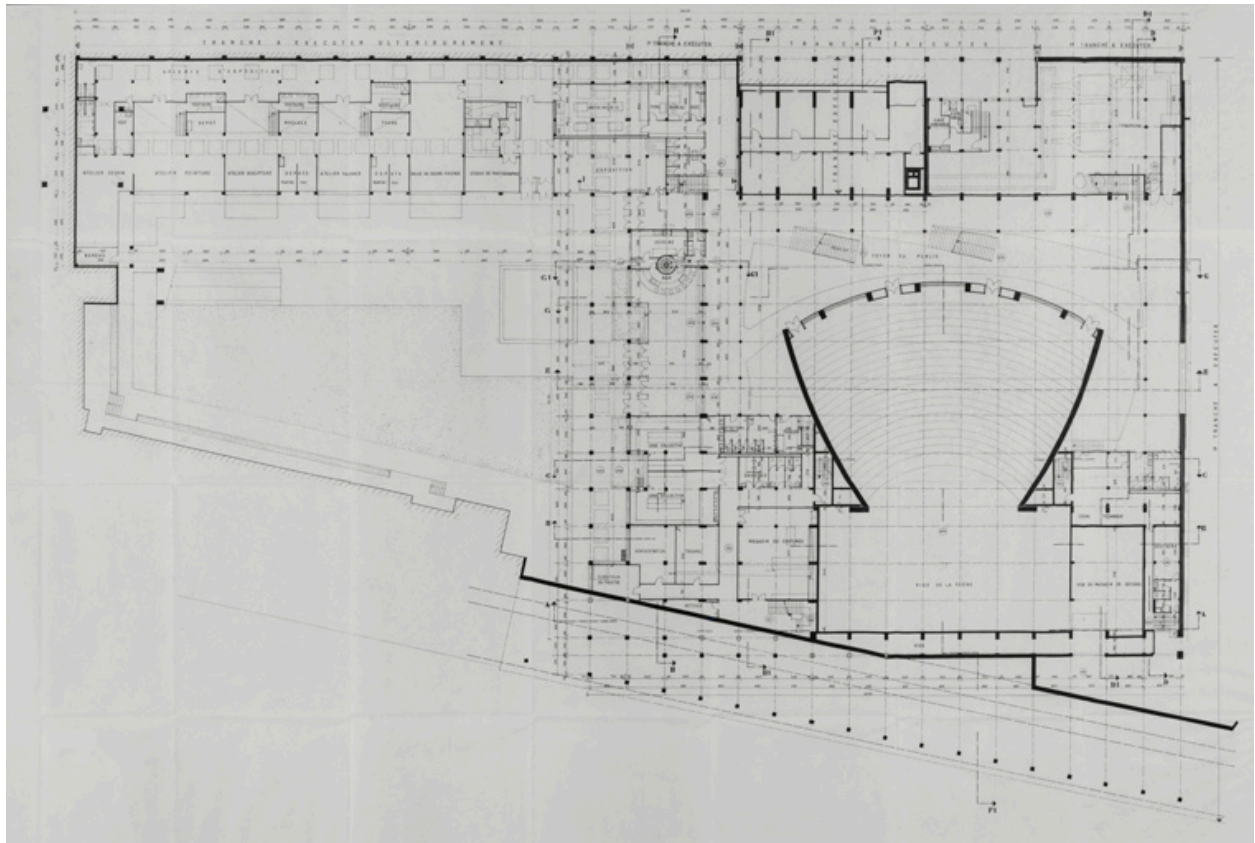
Nevers Centre municipal. Maison de la culture. 6. Plan d'exécution. Niveau jardin, parterre théâtre, loges collectives, ateliers artistes -150 -300 -350 -400. Octobre 1964, rect. novembre 1964.
