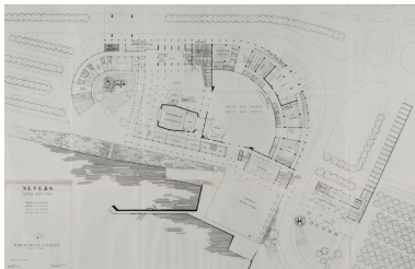
Nevers Centre municipal [...] 3. Plan du rez de chaussée. Novembre 1960-mars 1961. Phot. Pierre-Marie Barbe- Richaud, Autr. Max Guillaume, Autr. Henri Vauzelle IVR26_20245800791NUC4A
