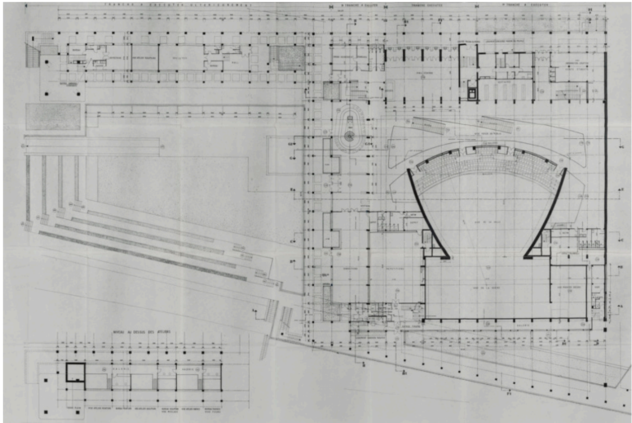
Nevers Centre municipal. Maison de la culture. 7. Plan d'exécution. Niveau rue, hall d'entrée, balcon théâtre, salle de répétitions, entrée garderie d'enfants +000 +100 +150. Octobre 1964, rect. novembre 1964.
