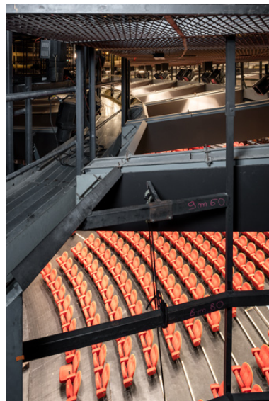
Maison de la culture, grande salle : charpente et passerelles techniques. Phot. Pierre-Marie Barbe-Richaud IVR26_20245800937NUC4A
