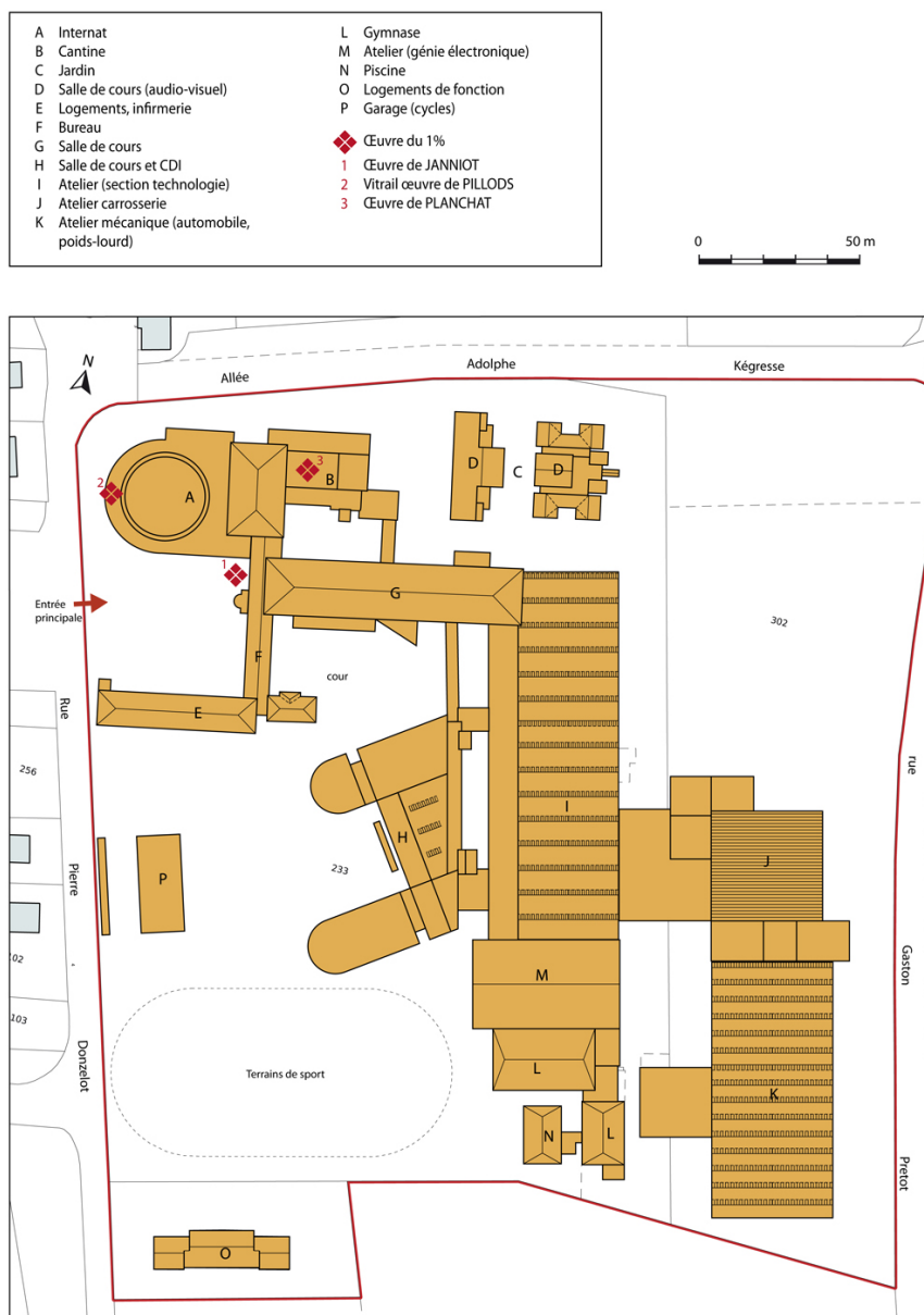
Plan-masse et de situation. Extrait du plan cadastral numérisé, sections BH et BL, échelle 1:1000.
