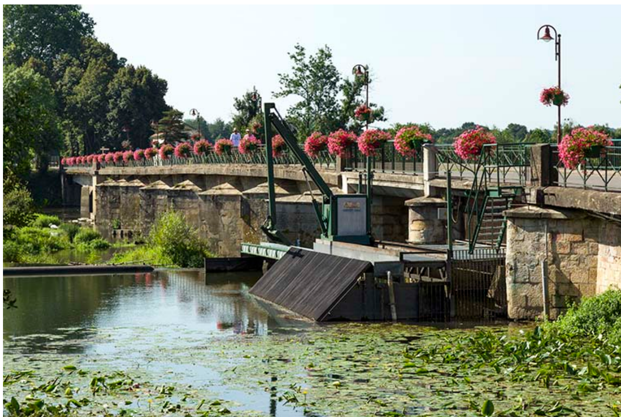
Le pont et la "portière" qui alimentait l'ancienne forge.
