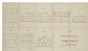
Fromagerie de Guyans-Vennes [Plans, coupes et élévations], s.d. [1923]. Phot. Sonia Dourlot IVR43_20152500540NUC4A
