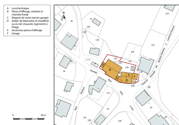
Plan-masse et de situation, section AB. Dess. Mathias Papigny IVR43_20142501915NUDA
