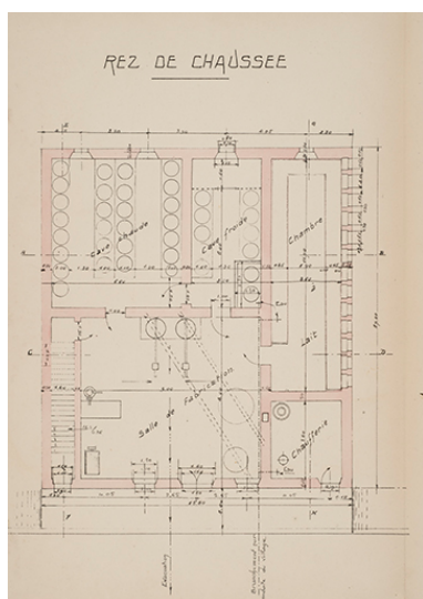
Fromagerie de Guyans-Vennes. Plan du rez-de-chaussée, s.d. [1923]. Phot. Sonia Dourlot IVR43_20152500488NUC4A
