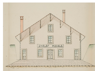
Fromagerie de Guyans-Vennes. Elévation de la façade antérieure, s.d. [1923]. Phot. Sonia Dourlot IVR43_20152500489NUC4A
