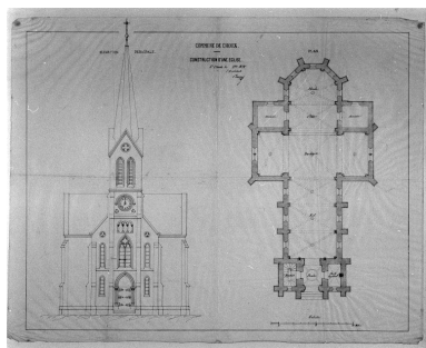
Commune de Choux. Construction d'une église [élévation principale et plan]. Phot. Jérôme Mongreville, Phot. Auguste Comoy IVR43_19943901384X
