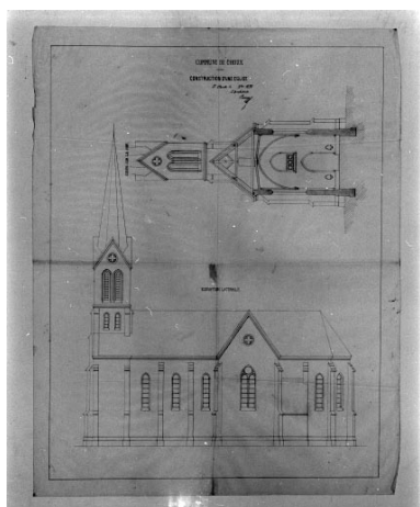
Commune de Choux. Construction d'une église [coupe sur la nef et élévation latérale]. Phot. Jérôme Mongreville, Phot. Auguste Comoy IVR43_19943901396X
