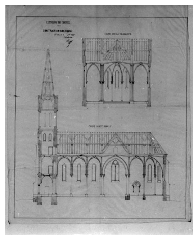
Commune de Choux. Construction d'une église [coupe sur le transept et coupe longitudinale]. Phot. Jérôme Mongreville, Phot. Auguste Comoy IVR43_19943901387X
