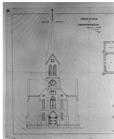
Commune de Choux. Construction d'une église [détail de l'élévation principale]. Phot. Jérôme Mongreville, Phot. Auguste Comoy IVR43_19943901388X
