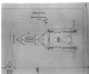
Commune de Choux. Construction d'une église [détail de la coupe sur la nef]. Phot. Jérôme Mongreville, Phot. Auguste Comoy IVR43_19943901395X
