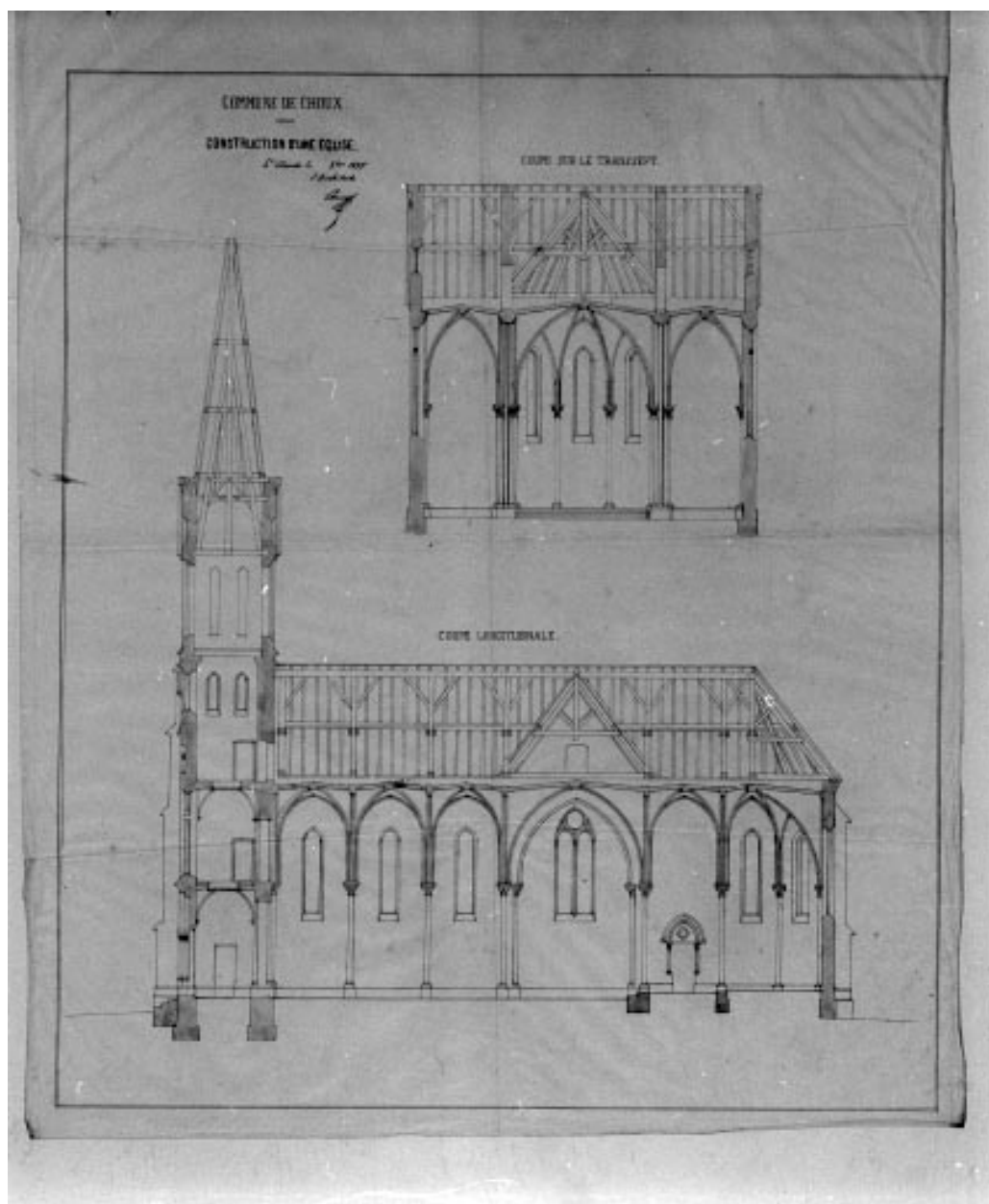
Commune de Choux. Construction d'une église [coupe sur le transept et coupe longitudinale].
