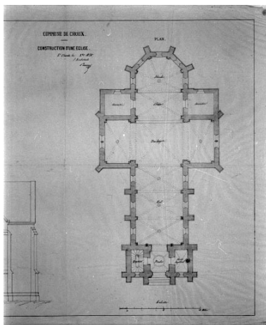
Commune de Choux. Construction d'une église [détail]. Phot. Jérôme Mongreville, Phot. Auguste Comoy IVR43_19943901383X
