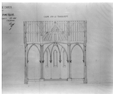
Commune de Choux. Construction d'une église [détail de la coupe sur le transept]. Phot. Jérôme Mongreville, Phot. Auguste Comoy IVR43_19943901389X
