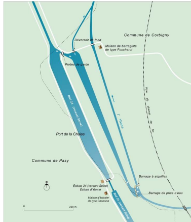
Carte schématique de la prise d'eau de la Chaise. Dess. Alain Morelière IVR26_20145800016NUDA
