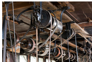
Arbre de transmission secondaire de la rangée centrale (au premier plan) et arbre principal (à l'arrière-plan).
