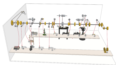
Le système de transmission par courroies. Dess. Mathias Papigny IVR43_20172501240NUDAQ
