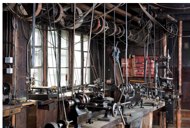
Machines de la rangée centrale et transmissions. Phot. Sonia Dourlot
