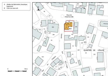
Plan-masse et de situation. Extrait du plan cadastral, 2015, section AE. Dess. Mathias Papigny IVR43_20152500670NUDA
