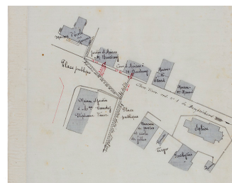
Chemin vicinal ordinaire n° 1 de Damprichard au Russey. Projet de construction d'aqueducs dans la traverse du village à Charquemont sur une longueur de [-] mètres. Plan d'ensemble, 4 octobre 1898. Phot. Sonia Dourlot, Autr. Bourquin IVR43_20142501731NUC2A
