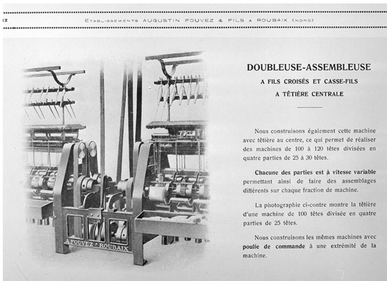
Doubleuse-assembleuse à fils croisés et casse-fils à têtère centrale.
