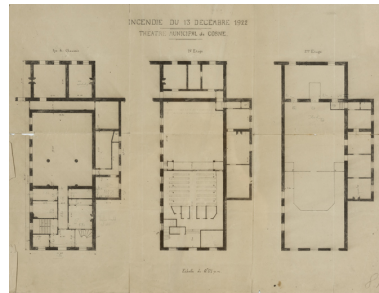
Incendie du 13 décembre 1922. Théâtre municipal de Cosne [plan du rez-de-chaussée et des deux étages]. S.d. [1922 ?]. Phot. Pierre-Marie Barbe-Richaud, Autr. auteur inconnu IVR26_20245800299NUC4A
