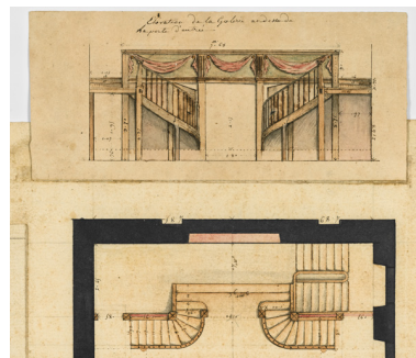
Projet de distribution de la salle de comédie de la ville de Cosne. [Rabat :] Elévation de la galerie au-dessus de la porte d'entrée. S.d. [1829]. Phot. Pierre-Marie Barbe-Richaud, Autr. Frossard IVR26_20245800283NUC4A
