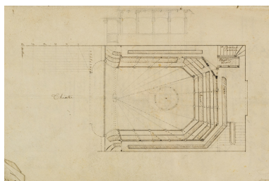
[Plan des loges et galeries]. S.d. [1830]. Phot. Pierre-Marie Barbe-Richaud, Autr. Frossard IVR26_20245800284NUC4A
