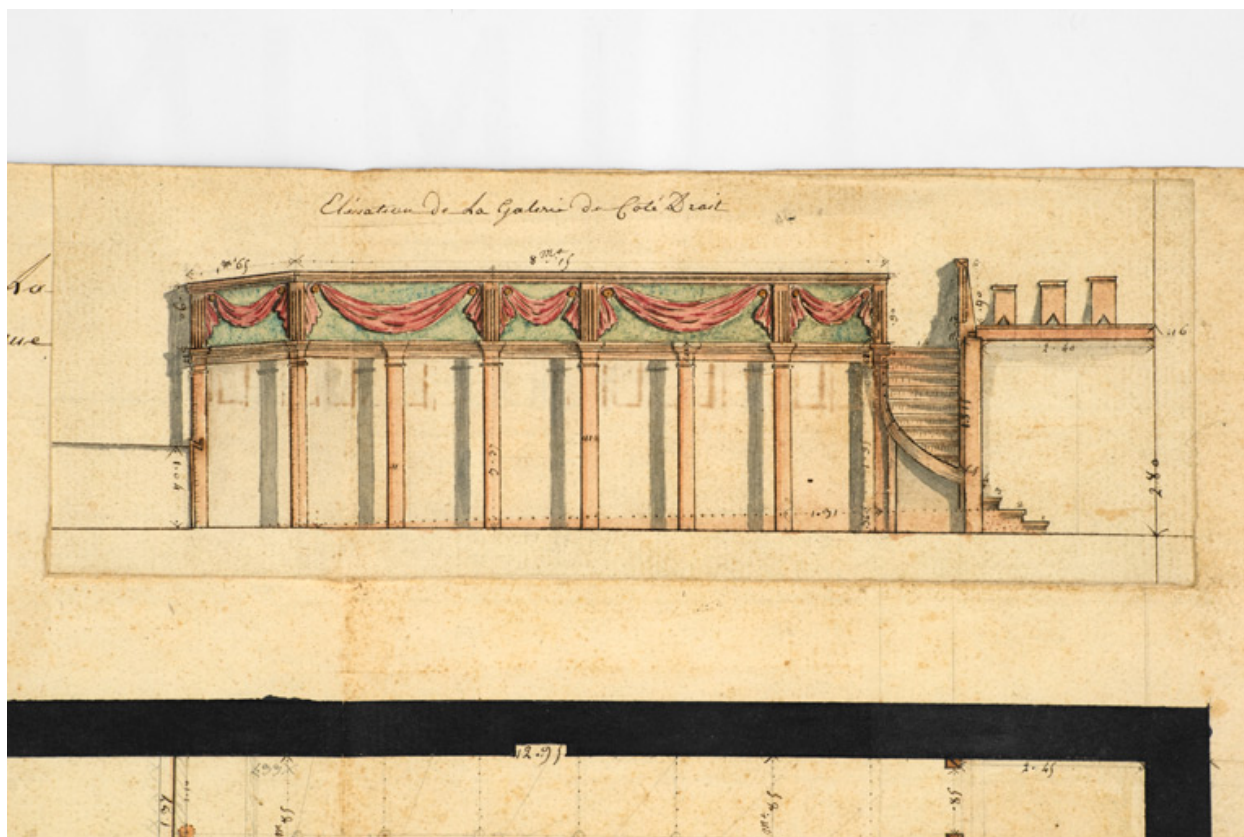
Projet de distribution de la salle de comédie de la ville de Cosne. [Rabat :] Elévation de la galerie du côté droit. S.d. [1829].
