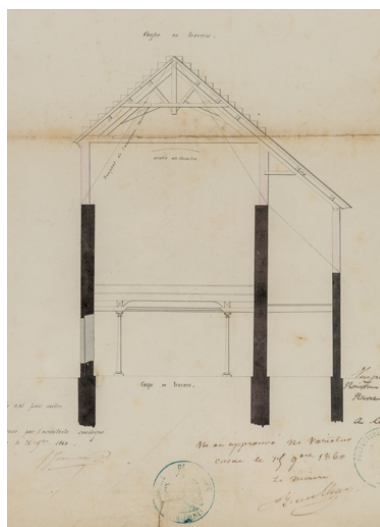
Ville de Cosne. Projet d'appropriation de l'ancien palais de justice et reconstruction de la charpente du comble. Coupe en travers. 15 novembre 1860. Phot. Pierre-Marie Barbe-Richaud, Autr. Ferdinand Jeaneau IVR26_20245800278NUC4A
