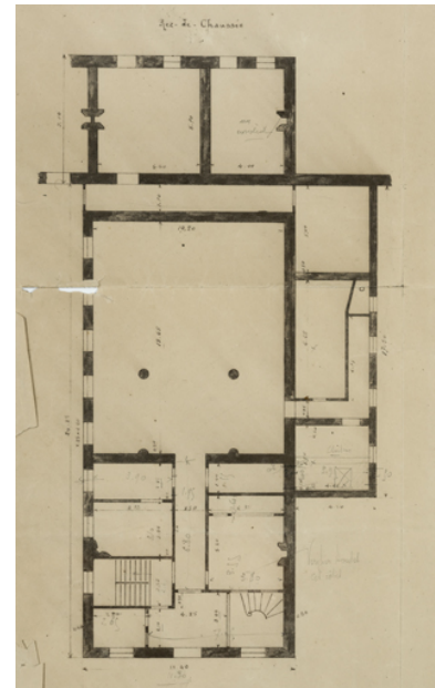
Incendie du 13 décembre 1922. Théâtre municipal de Cosne. Rez-de-chaussée. S.d. [1922 ?]. Phot. Pierre-Marie Barbe-Richaud, Autr. auteur inconnu IVR26_20245800297NUC4A
