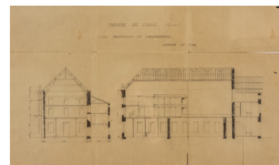
Théâtre de Cosne (Nièvre). Coupes transversale et longitudinale. S.d. [1922 ?]. Phot. Pierre-Marie Barbe-Richaud, Autr. auteur inconnu IVR26_20245800301NUC4A
