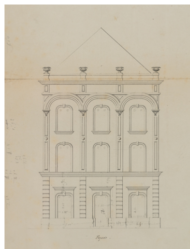
Ville de Cosne. Projet d'appropriation de l'ancien palais de justice et reconstruction de la charpente du comble. Façade. 15 novembre 1860. Phot. Pierre-Marie Barbe-Richaud, Autr. Ferdinand Jeaneau IVR26_20245800279NUC4A
