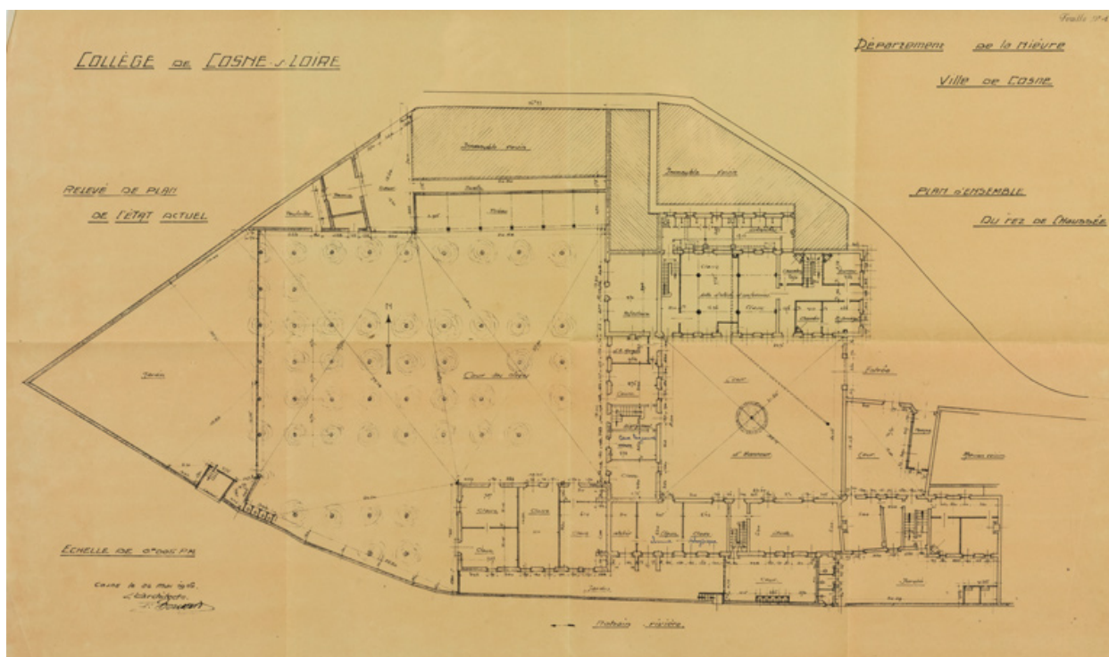
Collège de Cosne-s-Loire [état actuel]. Plan d'ensemble du rez de chaussée. 1936.
