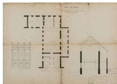
Ville de Cosne. Projet d'appropriation de l'ancien palais de justice et reconstruction de la charpente du comble. 15 novembre 1860. Phot. Pierre-Marie Barbe-Richaud, Autr. Ferdinand Jeaneau IVR26_20245800277NUC4A
