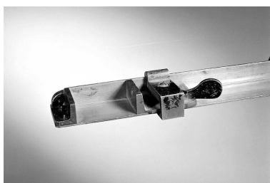
Blocage de l'équerre de l'un des composteurs métalliques : système à levier à axe vertical. Phot. Jérôme Mongreville IVR43_20023900083X
