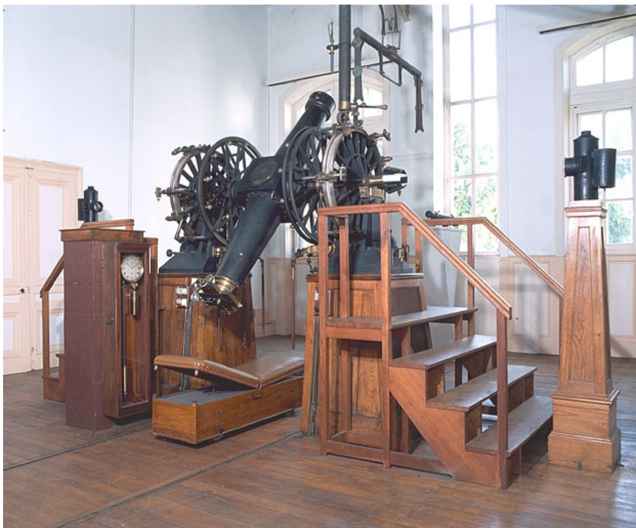
Observatoire (1883-1884), avenue de l'Observatoire : lunette méridienne utilisée pour "fabriquer l'heure".
