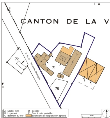
Plan-masse et de situation. Extrait du plan cadastral numérisé, 2008, section ZD, 1:2000 agrandi à 1:1000. Source : Direction générale des Finances Publiques - Cadastre ; mise à jour : 2008. Dess. André Céréza IVR43_20087000999NUDA
