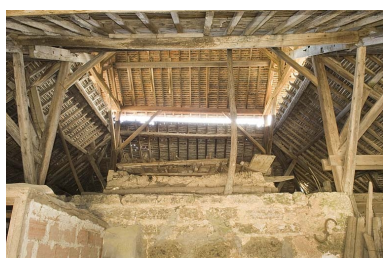
Vue intérieure du bâtiment du four. Massif maçonné. Phot. Jérôme Mongreville IVR43_20097000139NUC2A
