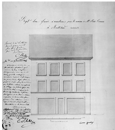
Projet d'une façade [... 6, rue Diemer-Duperret], 1846. Phot. Jérôme Mongreville IVR43_19862500499V
