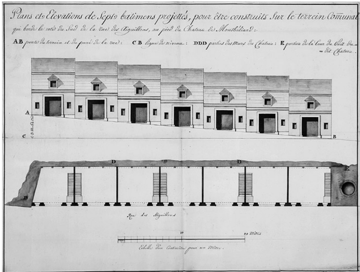
Plans et élévations de sept bâtimens projetés [... Rue du Château], fin 18e ou début 19e siècle.
