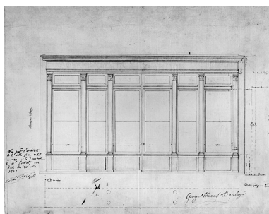
Projet de devanture [... 32, rue des Febvres], 1861. Phot. Jérôme Mongreville IVR43_19862500481V
