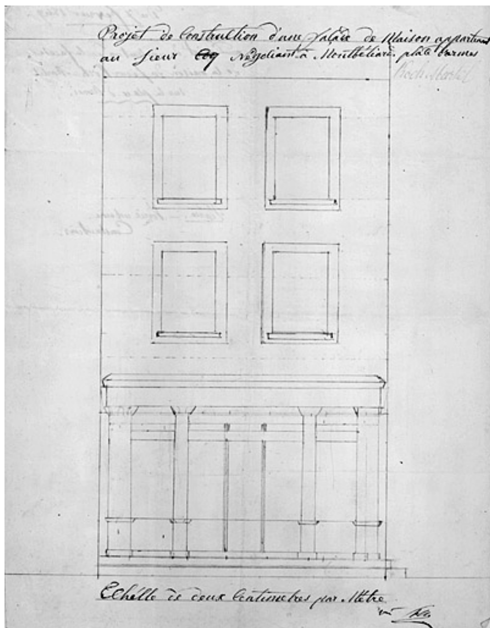
Projet de reconstruction d'une façade d'une maison [... 15, place Denfert-Rochereau], 1849.
