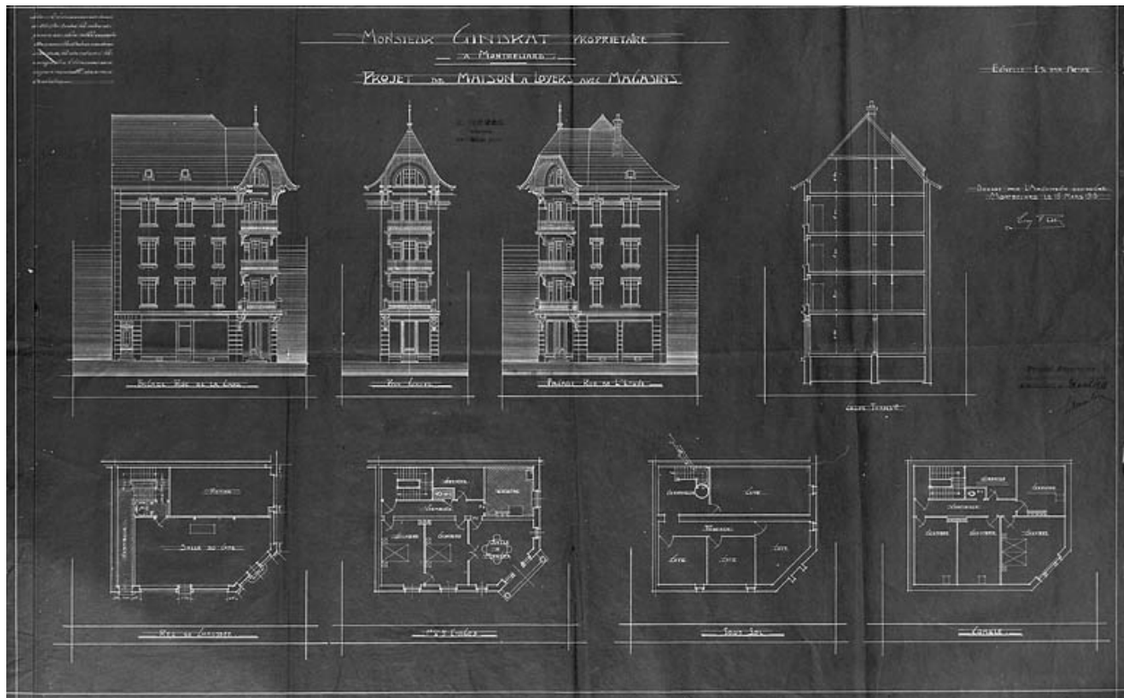
Projet de maison à loyers [... 33bis, avenue des Alliés], 1913.
