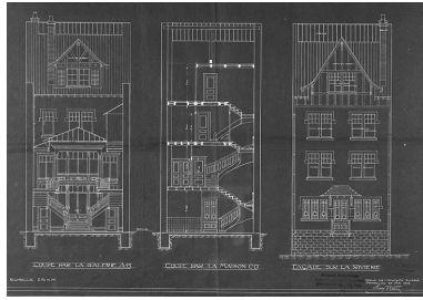
Projet d'agrandissement du magasin de Jules Jenn, rue Cuvier. Elévations et coupe transversale du deuxième corps de bâtiment, 1914. Phot. Yves Sancey, Autr. Eugène (architecte) NEPASUTILISERReess IVR43_19872500395V
