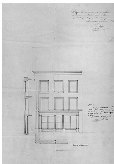
Projet de reconstruction d'une façade [... 16, rue du Général-Leclerc], 1863. Phot. Jérôme Mongreville IVR43_19862500489V
