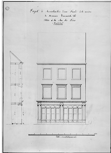
Projet [non réalisé] de reconstruction d'une façade [... 31, rue des Febvres], 1851. Phot. Jérôme Mongreville IVR43_19862500502V
