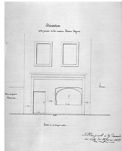
Elévation de la façade de la maison Eléonore Ségur [projet d'une ouverture de boutique. 5, rue Cuvier], 1866. Phot. Jérôme Mongreville IVR43_19862500503V
