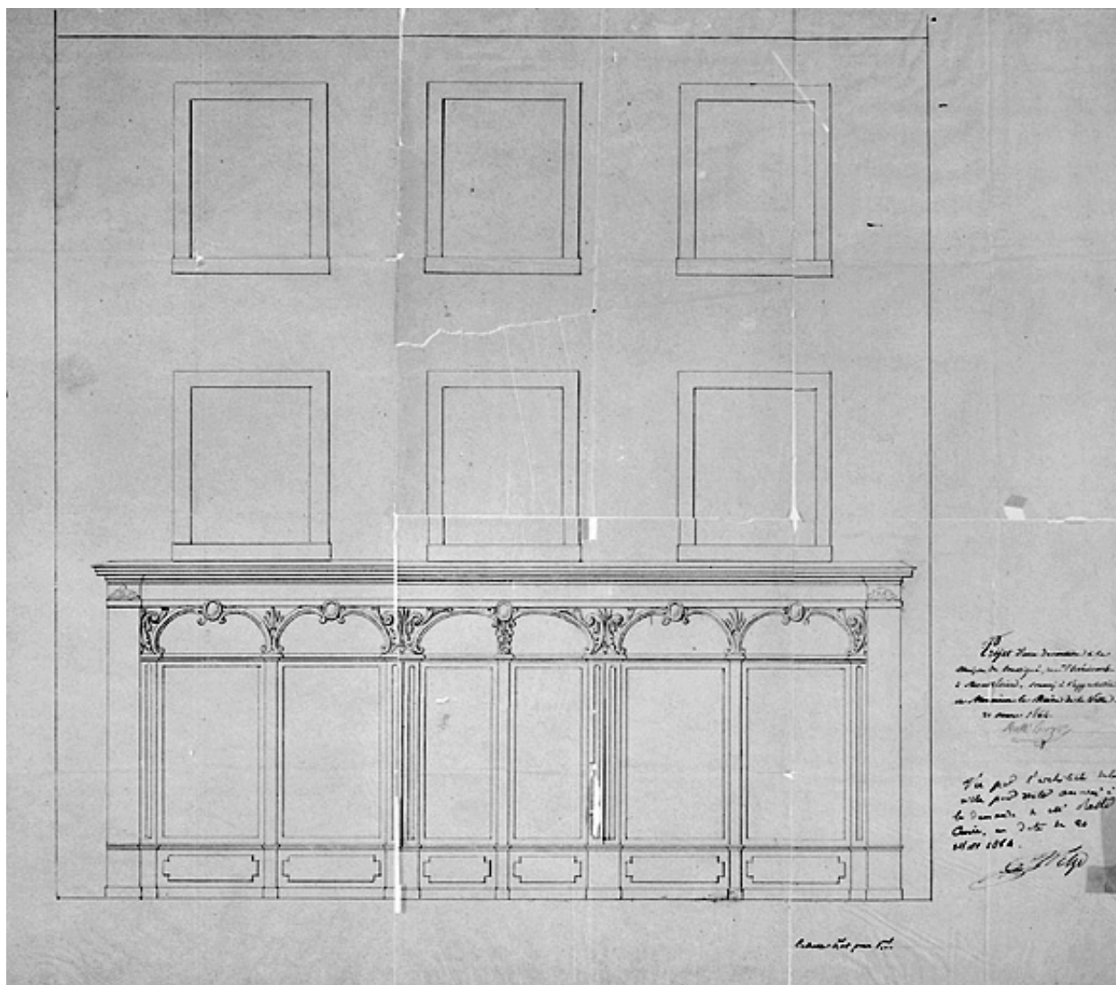
Projet d'une devanture [... 1, rue du Général-Leclerc], 1864.
