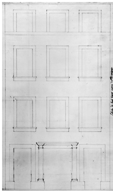
Projet de reconstruction de la façade d'une maison [... Rue Georges-Clémenceau], 1829. Phot. Jérôme Mongreville IVR43_19862500478V
