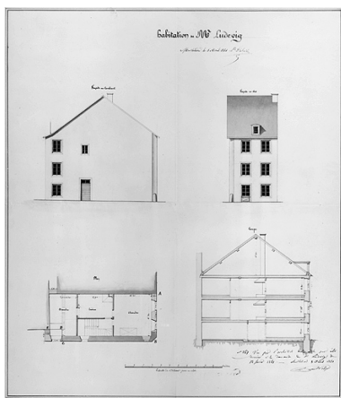
Habitation de M. Ludevig [3, rue du Bourg Vauthier], 1861. Phot. Jérôme Mongreville, Autr. L. Flubaker IVR43_19862500486V
