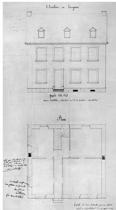
Maison d'habitation à construire rue de la Tuilerie [... Rue Saint-Georges], 1865.
