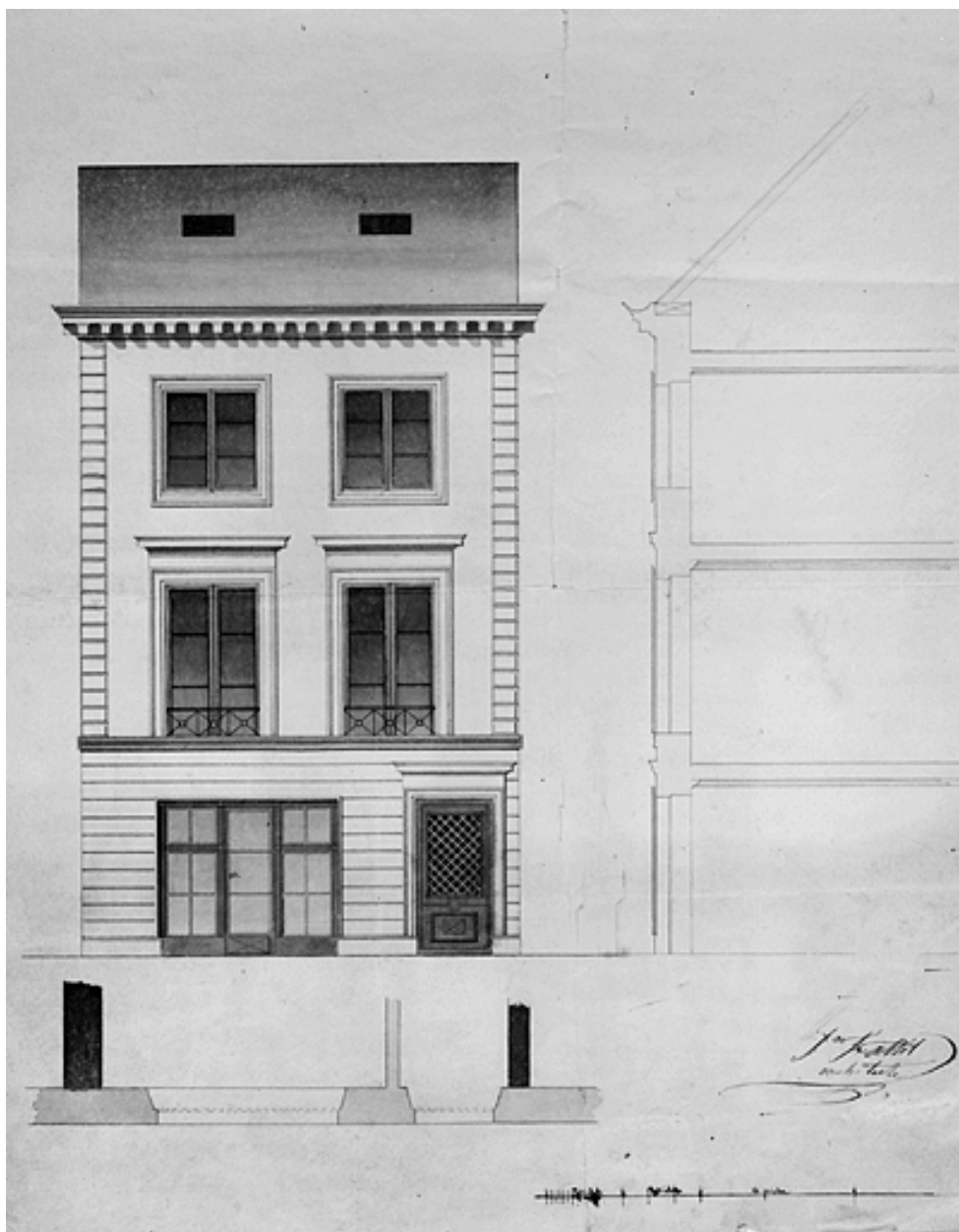
Plan de la maison [coupe et élévation de la façade] de Mme Veuve Megnin-Fallot [... 55, rue du Faubourg], vers 1840-1850.
