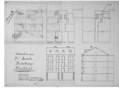
Construction pour M. Journet [... 40, rue Georges-Clémenceau], 1914. Phot. Yves Sancey, Autr. Léon (architecte) NEPASUTILISERRossel IVR43_19872500066V
