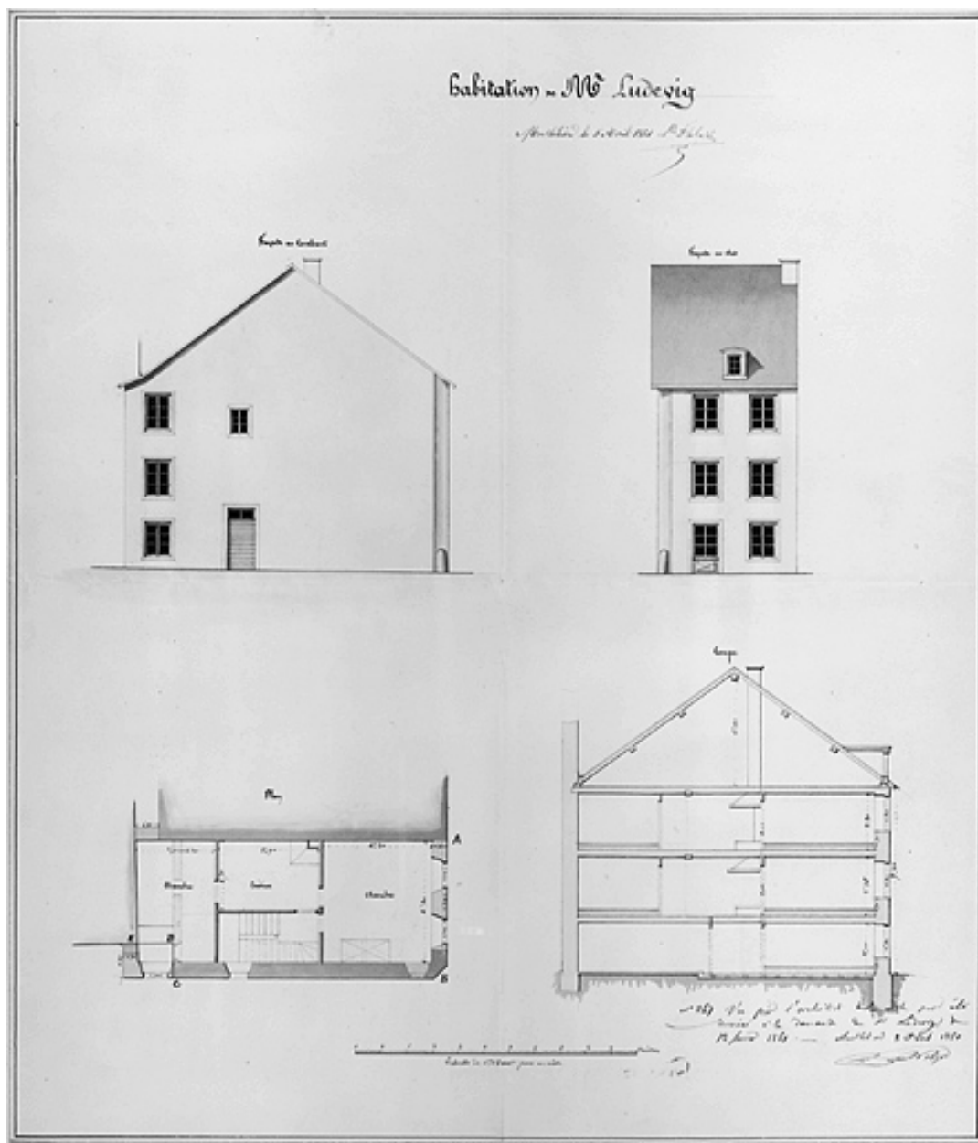
Habitation de M. Ludevig [3, rue du Bourg Vauthier], 1861.
