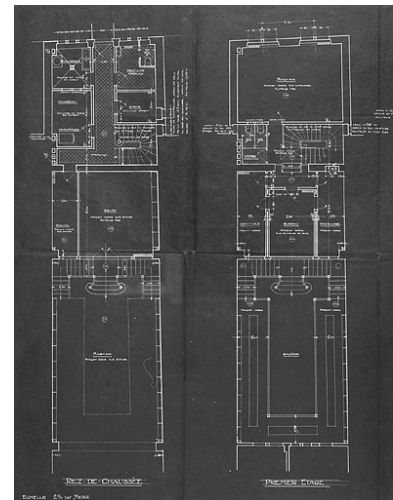
Projet d'agrandissement du magasin de Jules Jenn, rue Cuvier. Plans du rez-de-chaussée et du premier étage, 1914. Phot. Yves Sancey, Autr. Eugène (architecte) NEPASUTILISERReess IVR43_19872500397V
