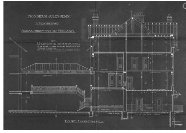
Projet d'agrandissement du magasin de Jules Jenn, rue Cuvier. Coupe longitudinale du deuxième corps de bâtiment, 1914. Phot. Yves Sancey, Autr. Eugène (architecte) NEPASUTILISERReess IVR43_19872500396V
