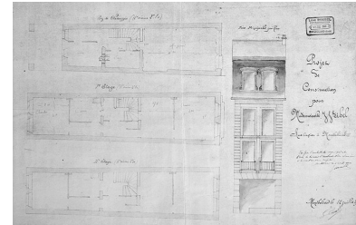
Projet de construction [... 14 (?), rue Cuvier], 1909. Phot. Jérôme Mongreville, Autr. Léon (architecte) NEPASUTILISERRossel IVR43_19872500065V
