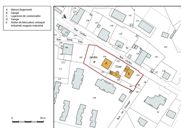
Plan-masse et de situation. Extrait du plan cadastral, 2018, section AP. Dess. Bertrand Turina IVR43_20202500262NUDA
