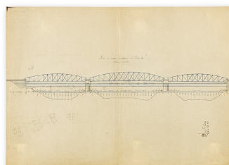
Elévation d'aval du pont métallique de Fleurville. 1899. Phot. Thierry Kuntz IVR26_20197100726NUC4A
