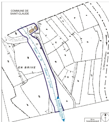
Plan-masse et de situation. Extrait du plan cadastral informatisé, 2006, section C, échelle 1:1250. Dess. André Céréza IVR43_20073900286NUDA
