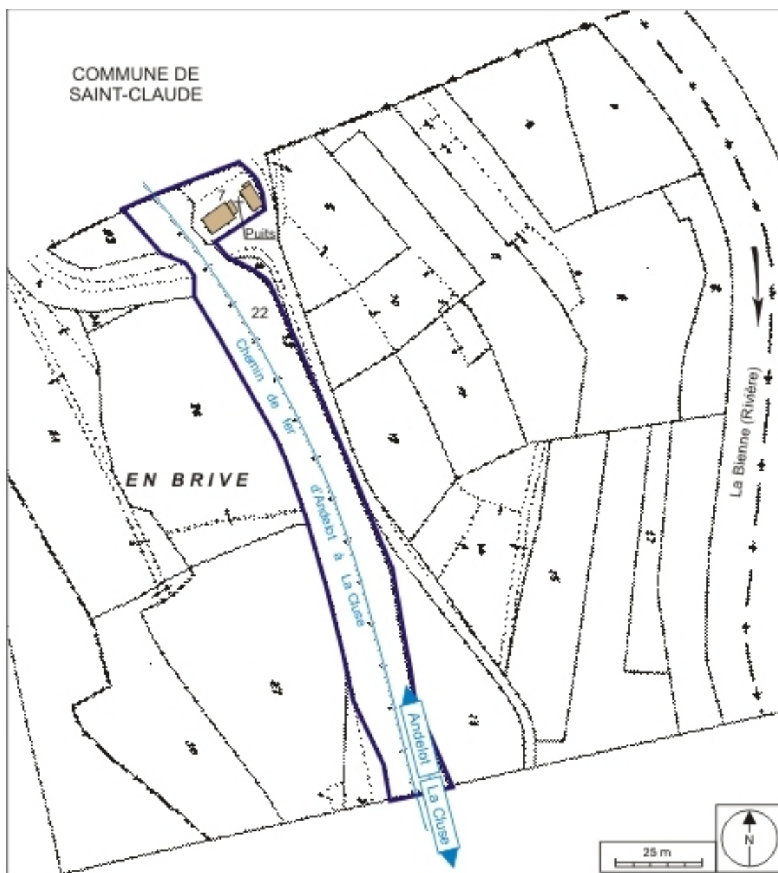
Plan-masse et de situation. Extrait du plan cadastral informatisé, 2006, section C, échelle 1:1250.
