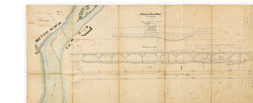
Dessins du pont de Seurre à joindre à notre rapport en date de ce jour sur la demande de diverses chambres de Commerce. 24 septembre 1856.
