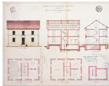
Projet de construction d'une maison commune : plan, coupe et dispositions des étages (1861). Phot. Jérôme Mongreville, Autr. Claude François Charles Dodelier IVR43_20177001166NUC4A
