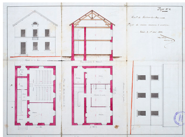
1er projet délivré pour la construction d'une maison commune. Phot. Jérôme Mongreville, Autr. Claude François Charles Dodelier IVR43_20177001168NUC4A
