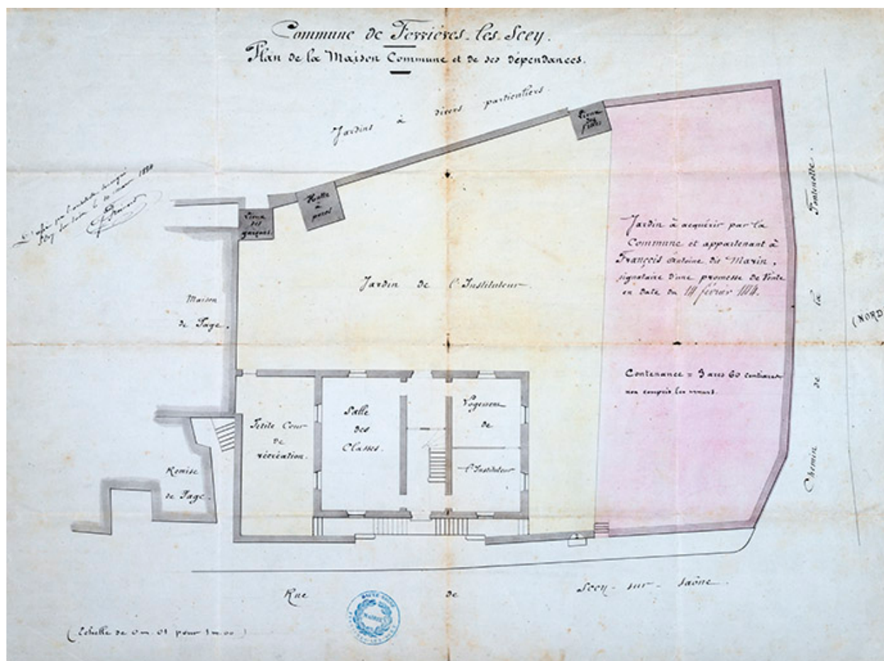
Plan de la maison commune et de ses dépendances (1884).
