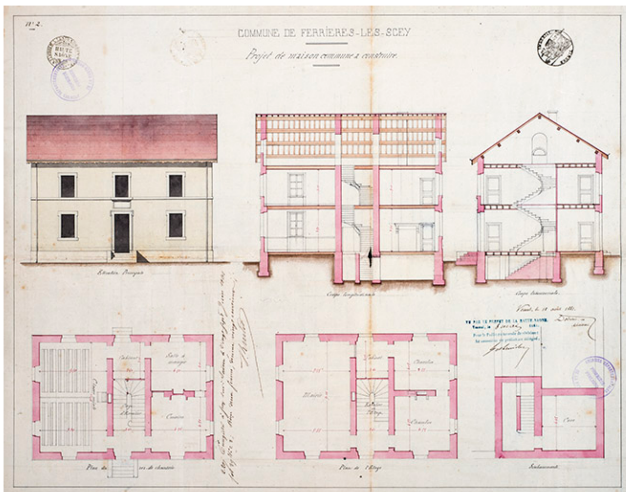
Projet de construction d'une maison commune : plan, coupe et dispositions des étages (1861).
