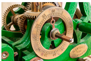
Détail, le cadran (vue de trois quarts). Phot. Jérôme Mongreville IVR43_20207000251NUC4A
