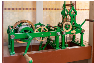
Vue du mécanisme avec ses manivelles. Phot. Jérôme Mongreville IVR43_20207000250NUC4A
