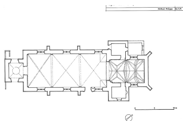
Plan au sol. Phot. Yves Sancey IVR43_19772500283V
